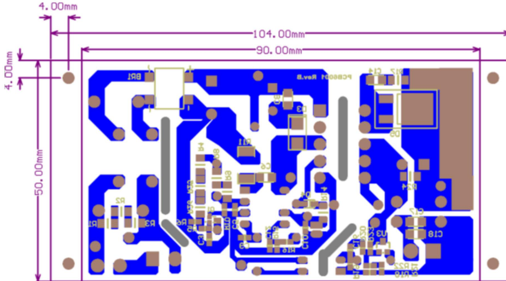
Bottom Layer
