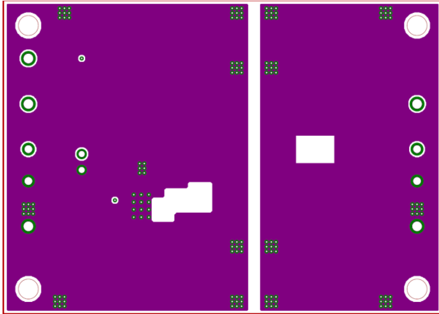
Middle Layer2 レイアウト
