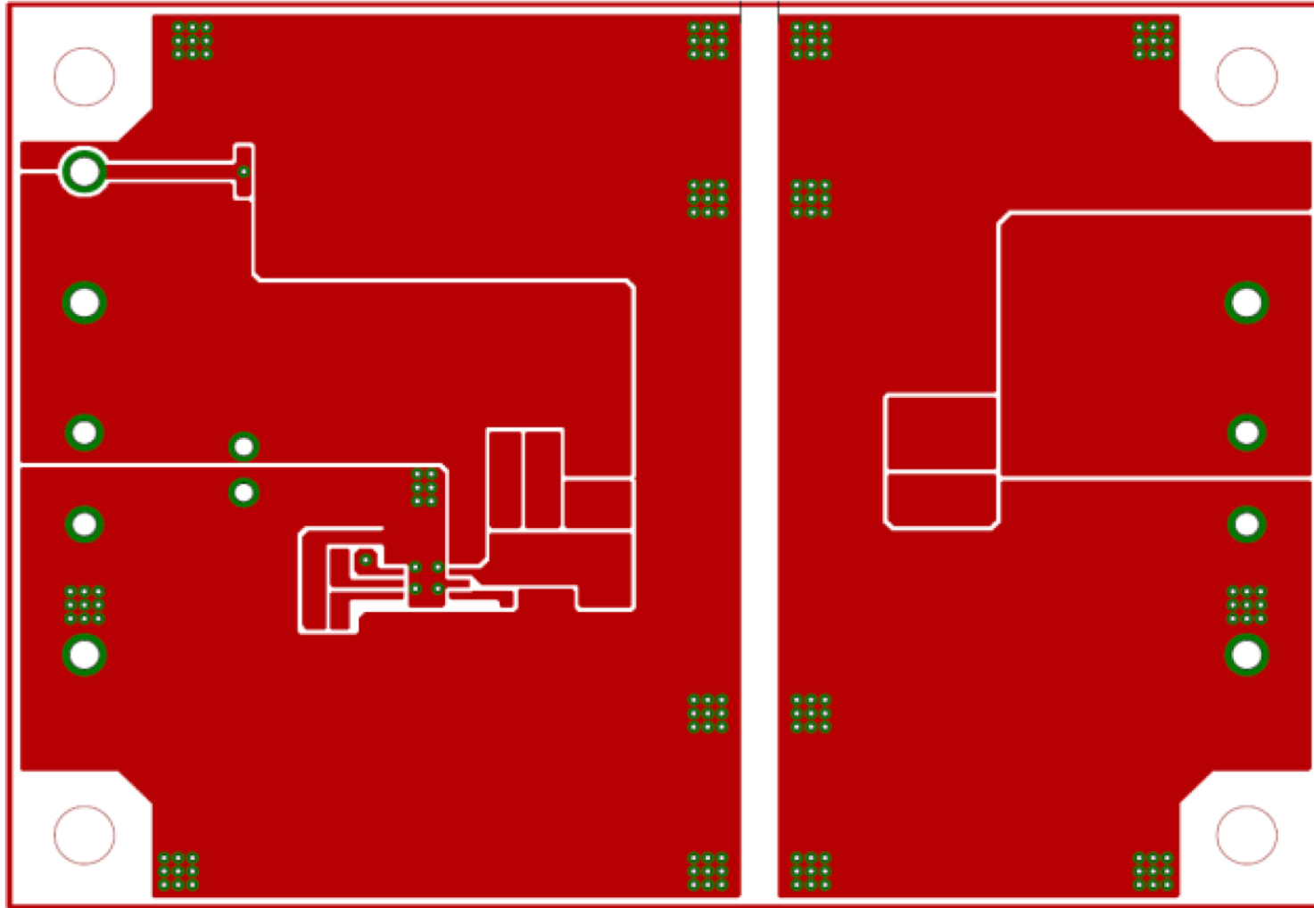
Top Layer レイアウト
