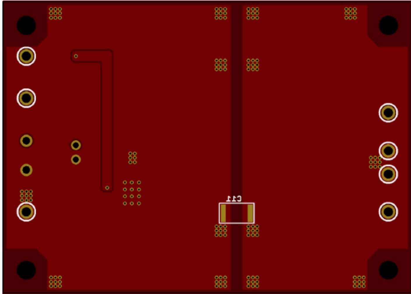
Bottom シルクスクリーン,レイアウト
