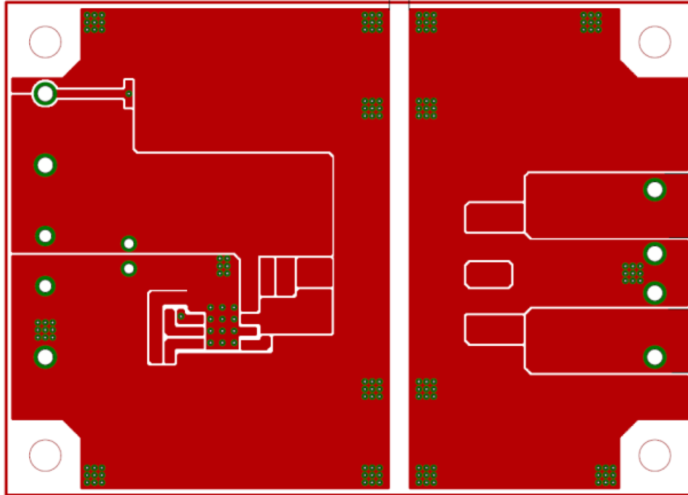
Top Layer レイアウト
