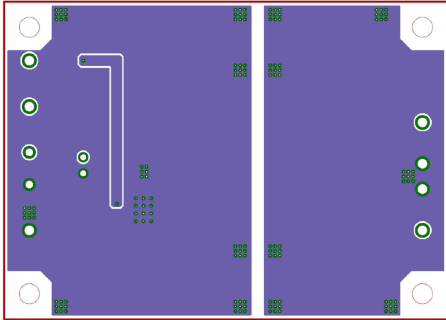
Bottom Layer レイアウト
