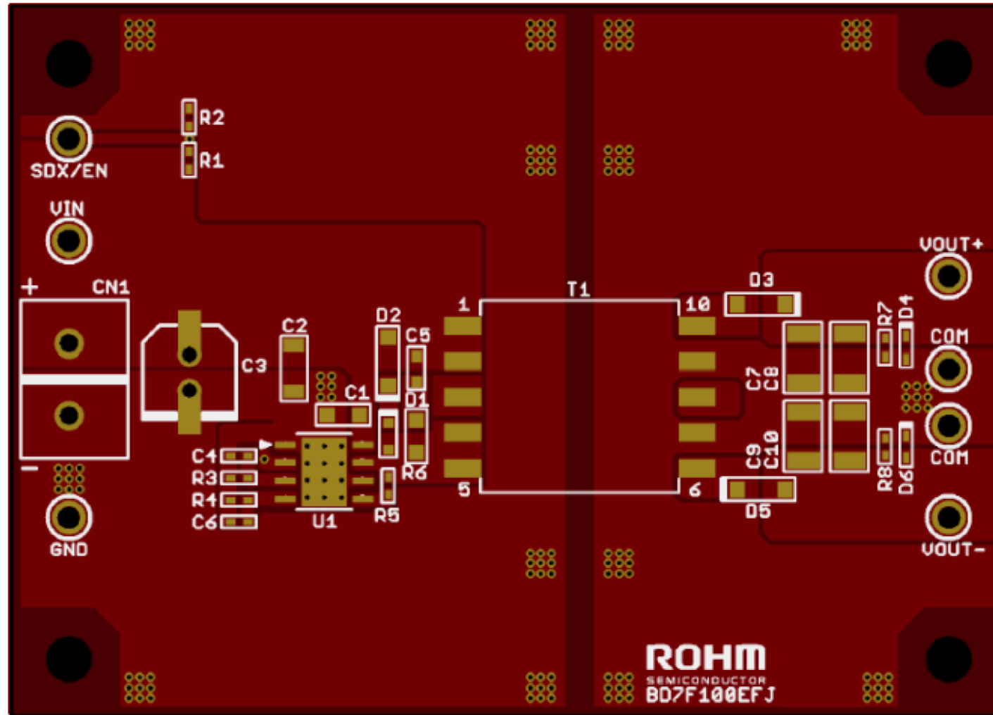
Top シルksクリーン,レイアウト
