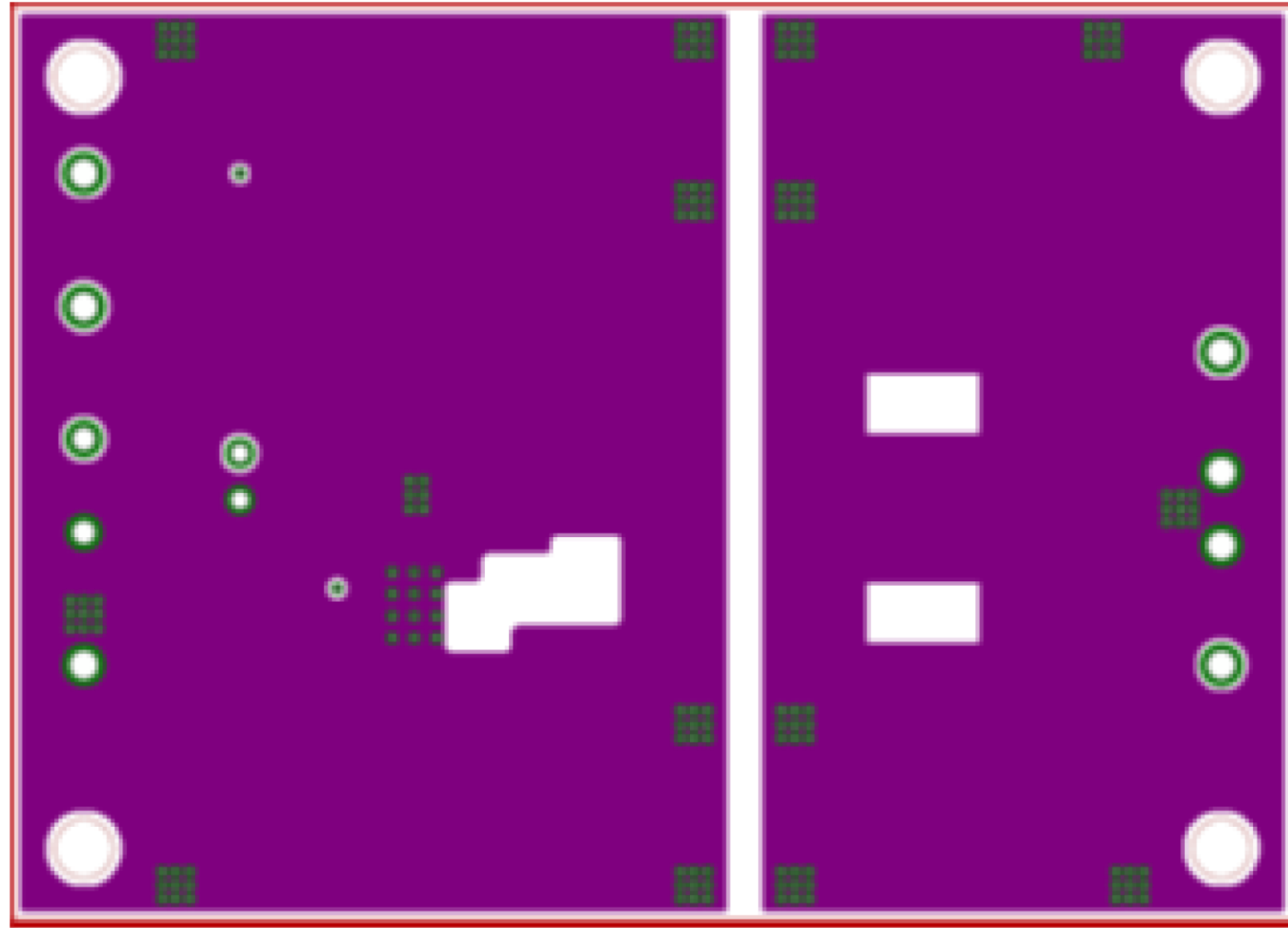
Middle Layer2 レイアウト
