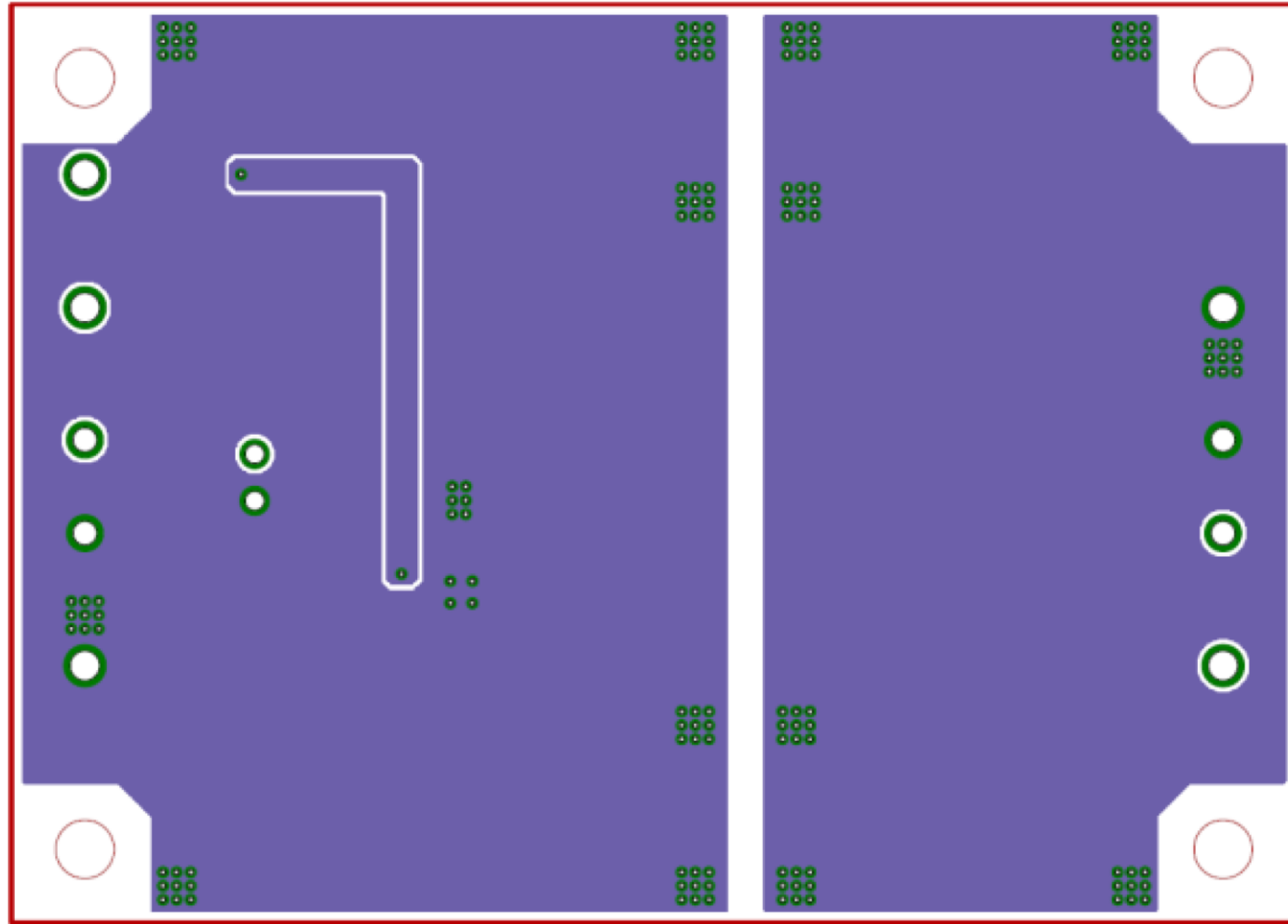
Bottom Layer レイアウト
