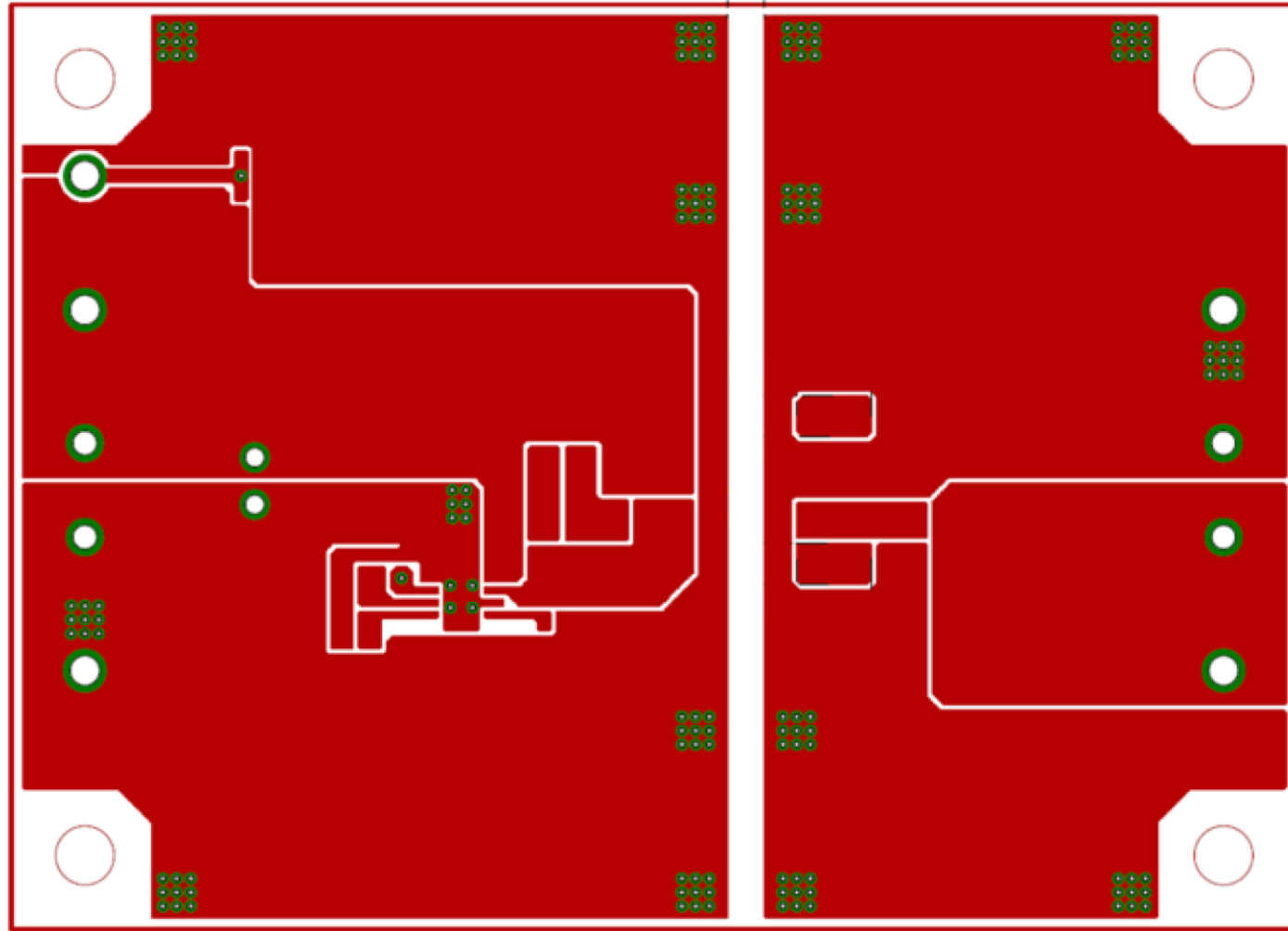
Top Layer レイアウト
