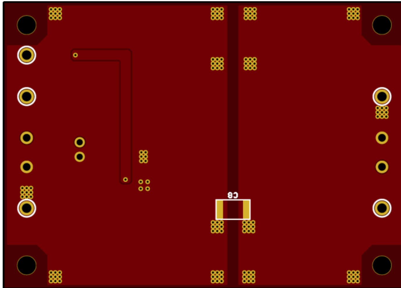
Bottom シルクスクリーン,レイアウト
