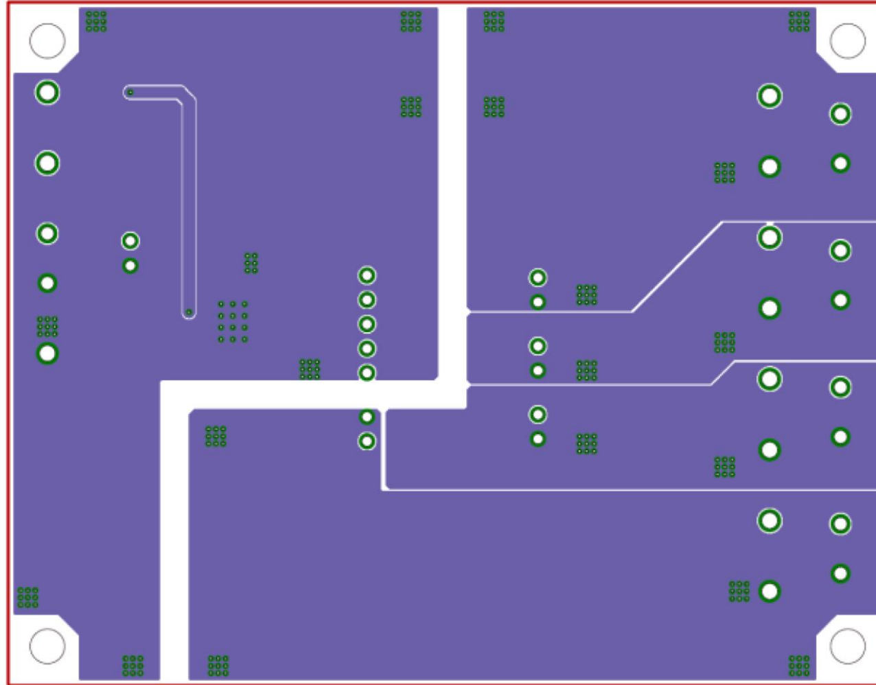
Bottom Layer レイアウト
