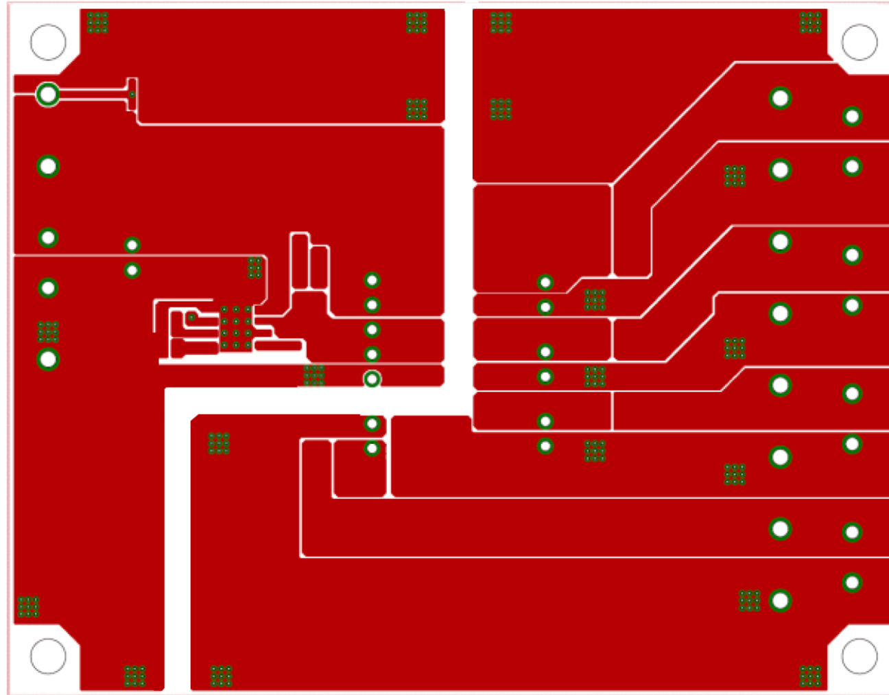
Top Layer レイアウト
