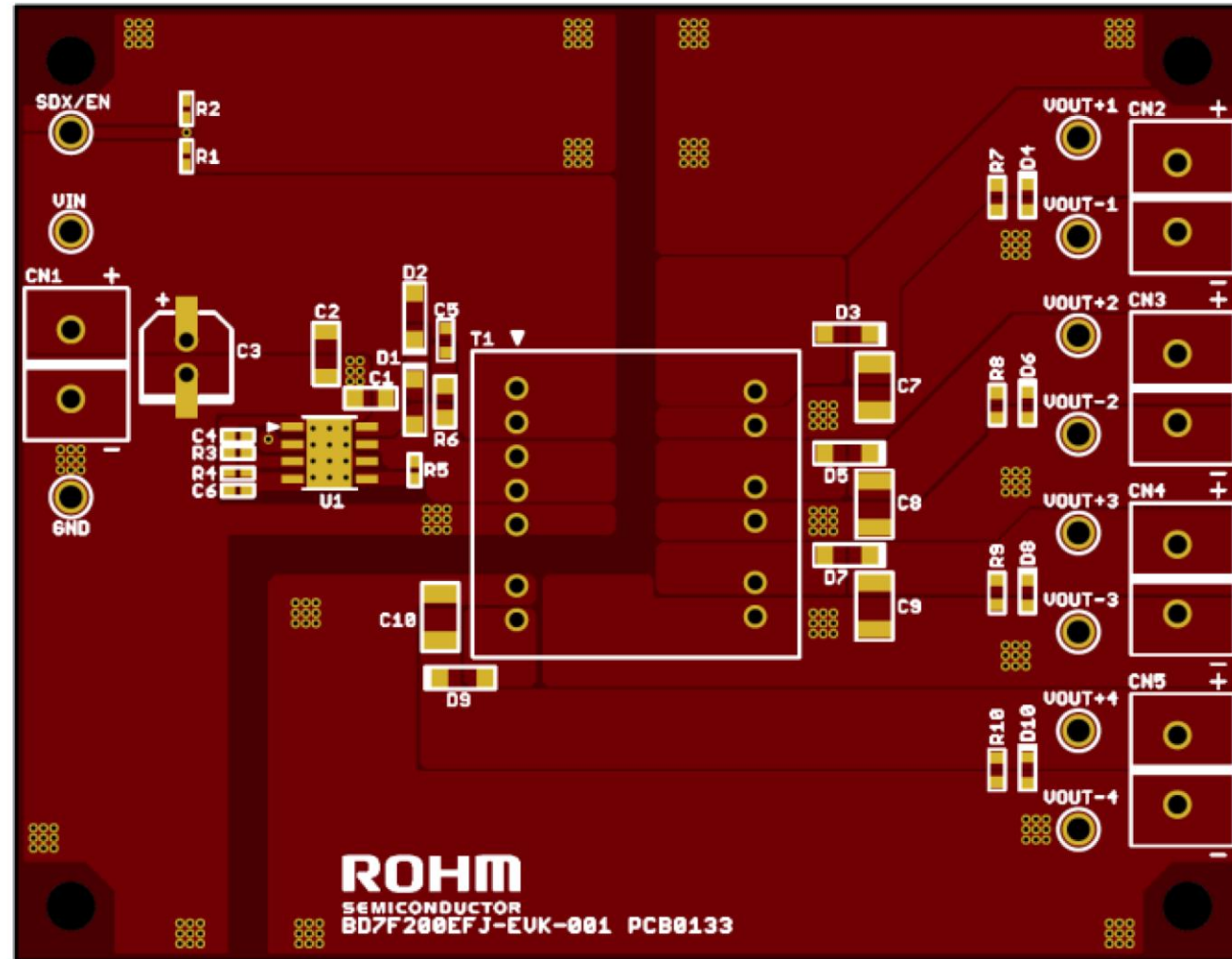
Top シルクスクリーン,レイアウト
