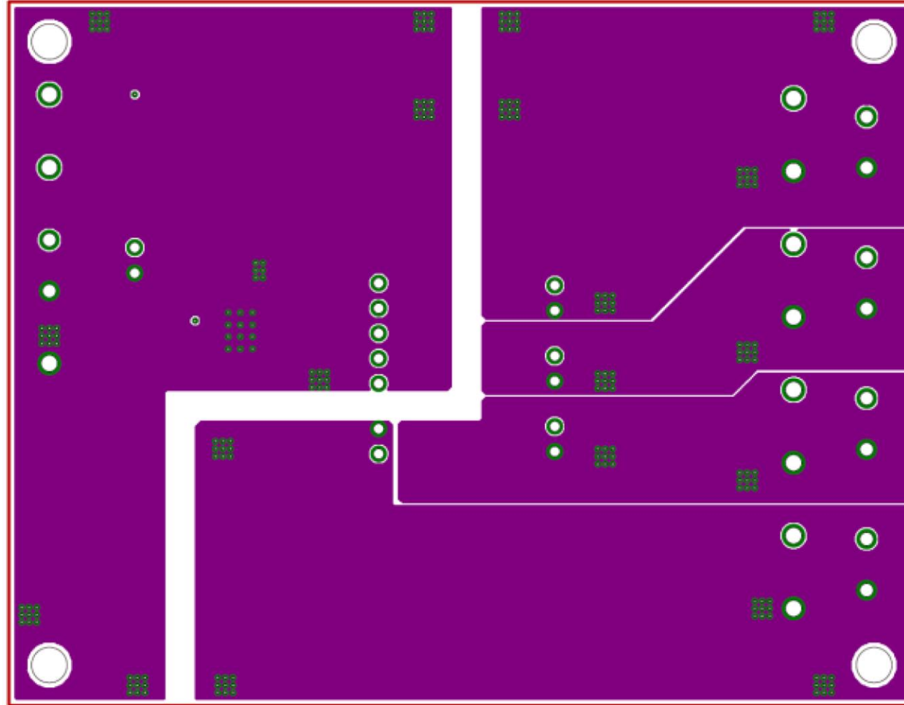
Middle Layer2 レイアウト
