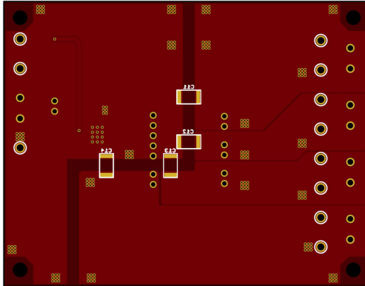
Bottom シルクスクリーン,レイアウト
