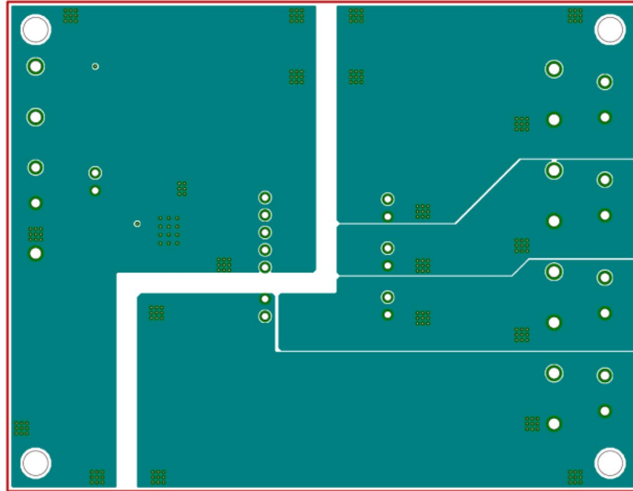
Middle Layer1 レイアウト
