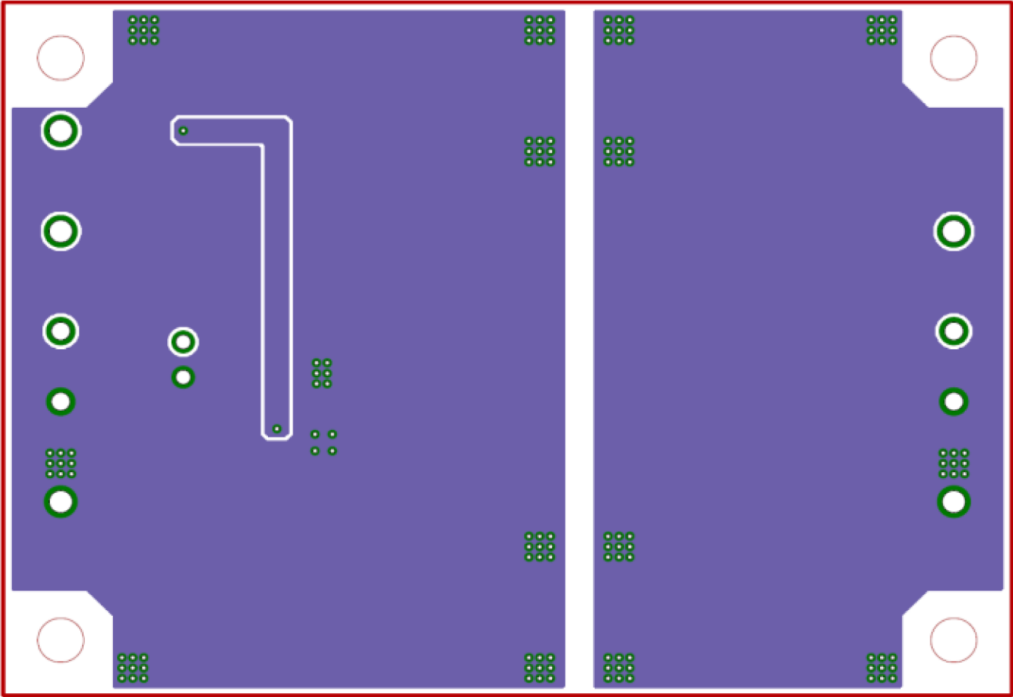
Bottom Layer レイアウト
