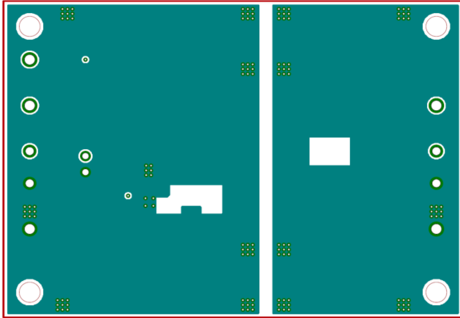
Middle Layer1 レイアウト
