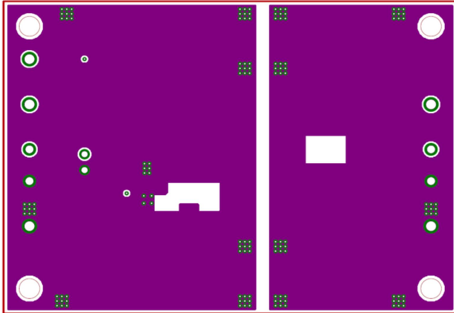
Middle Layer2 レイアウト
