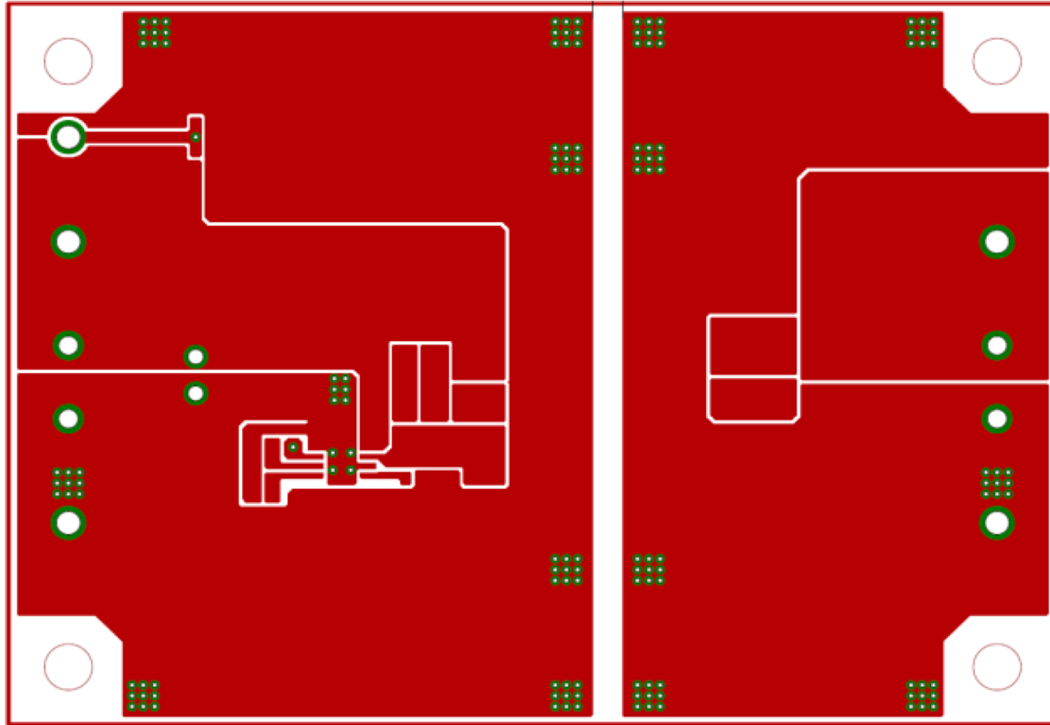
Top Layer レイアウト
