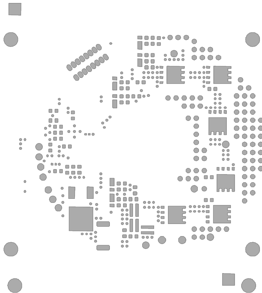
Bottom_Mask
