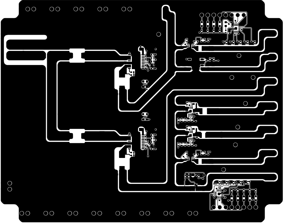
F_Cu
