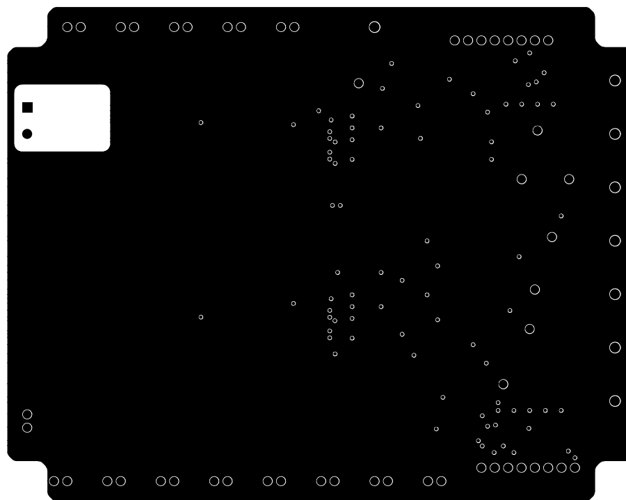
In1
