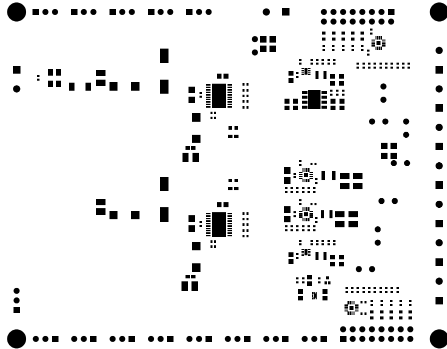
F_Mask
