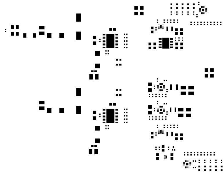
F_Paste
