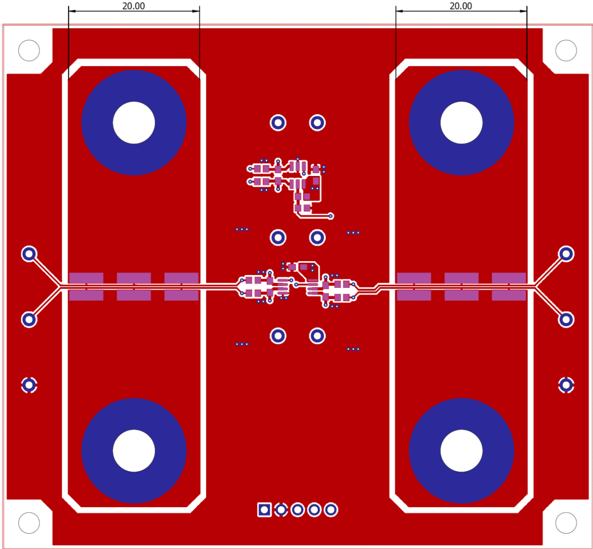
Top View Top Layer
