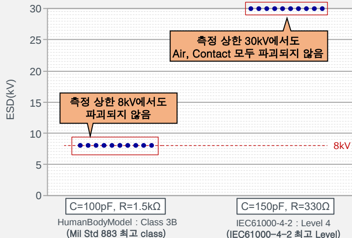
ESD 내성 데이터 (UDZV5.6B)
