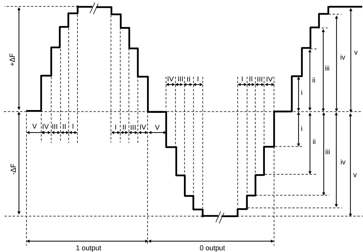
TX_FSK_POL ([DATA_SET1:B0 0x07(6)]) = 0b0 setting
