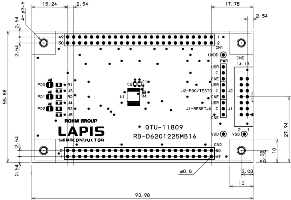
図 5. ML62Q1225 Reference Board 基板寸法図(TopView)
