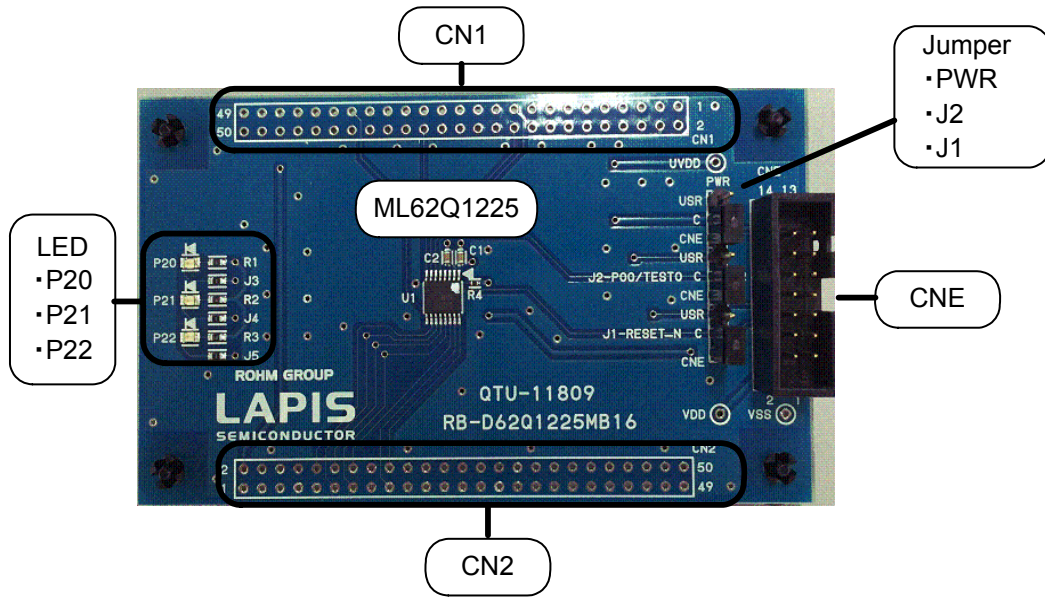
図 1. ML62Q1225 Reference Board 外観図
