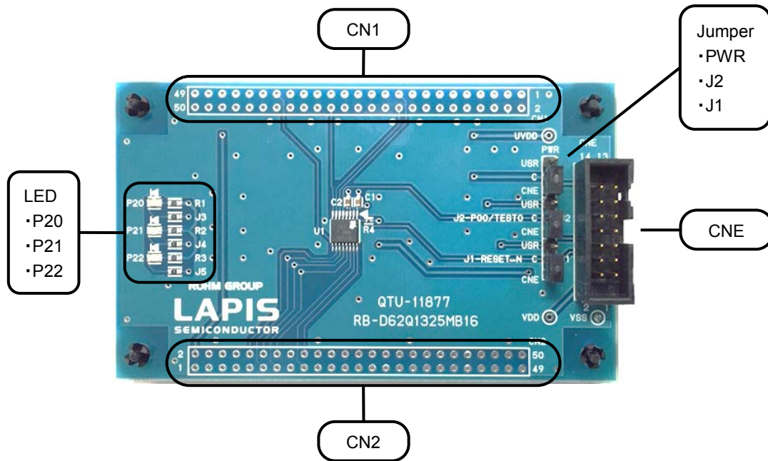
図 1 ML62Q1325 Reference Board 外観図
