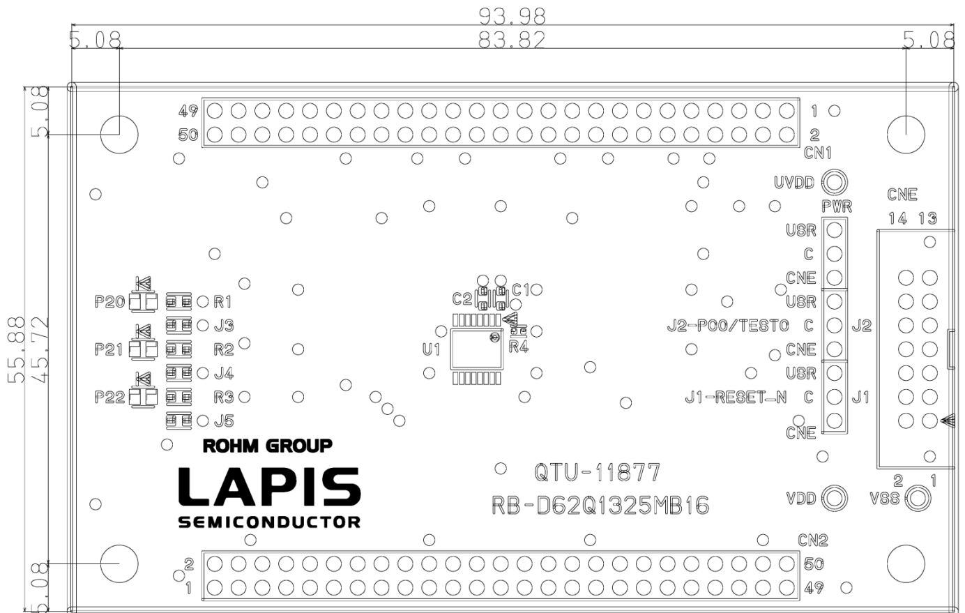
図 5 ML62Q1325 Reference Board 基板寸法図(TopView)
