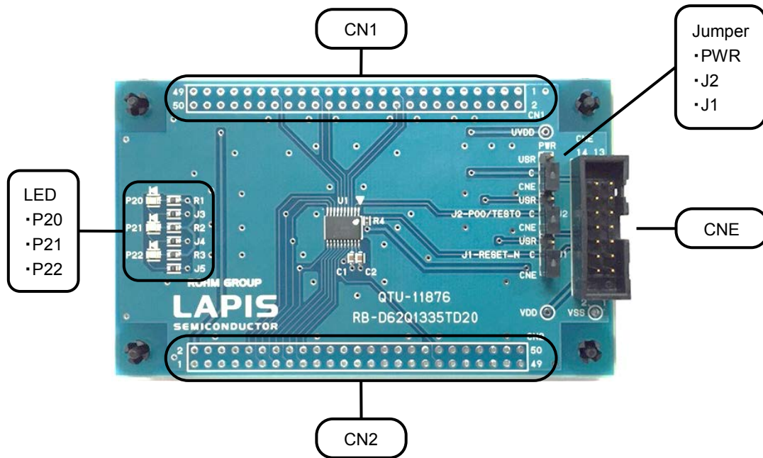
図 1 ML62Q1335 Reference Board 外観図
