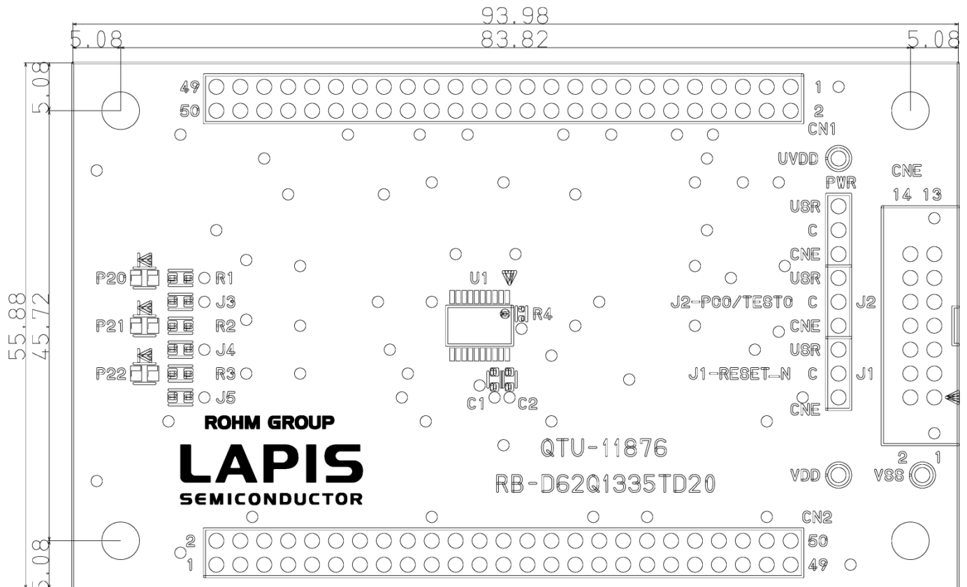
図 5 ML62Q1335 Reference Board 基板寸法図(TopView)
