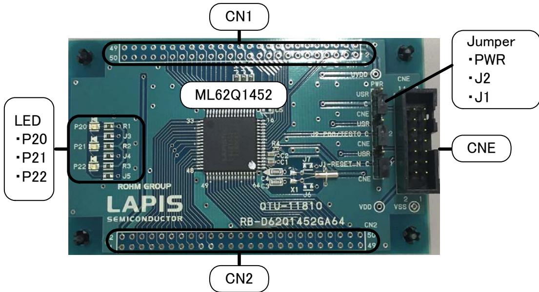
図 1. ML62Q1452 Reference Board 外観図
