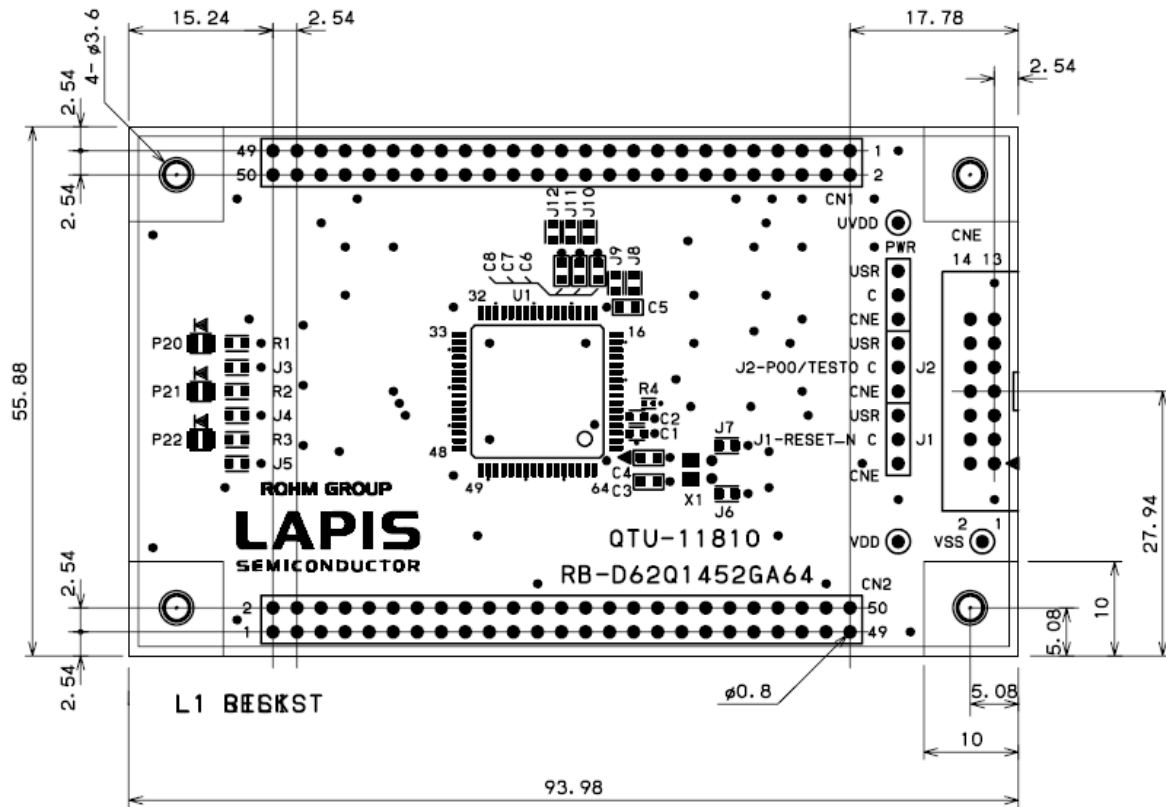
図 7. ML62Q1452 Reference Board 基板寸法図(TopView)
