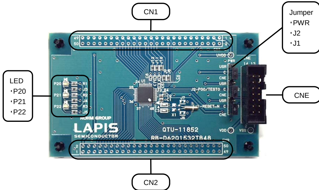
図 1 ML62Q1532 Reference Board 外観図
