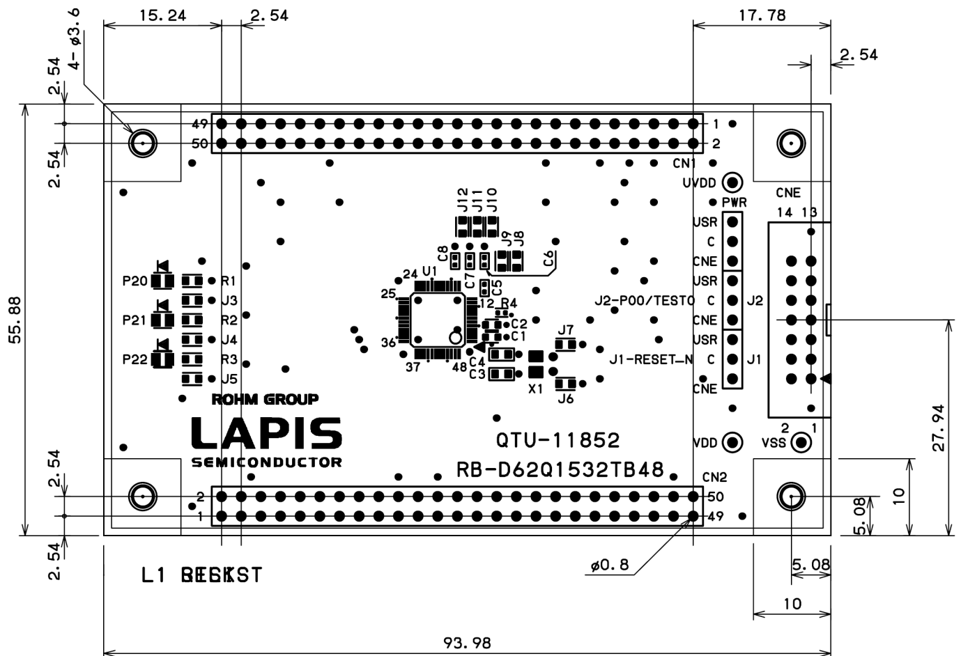
図 7 ML62Q1532 Reference Board 基板寸法図(TopView)
