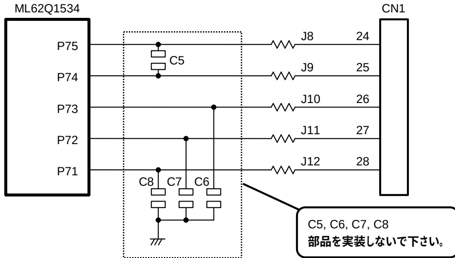
図 6 P75-P71 の回路
