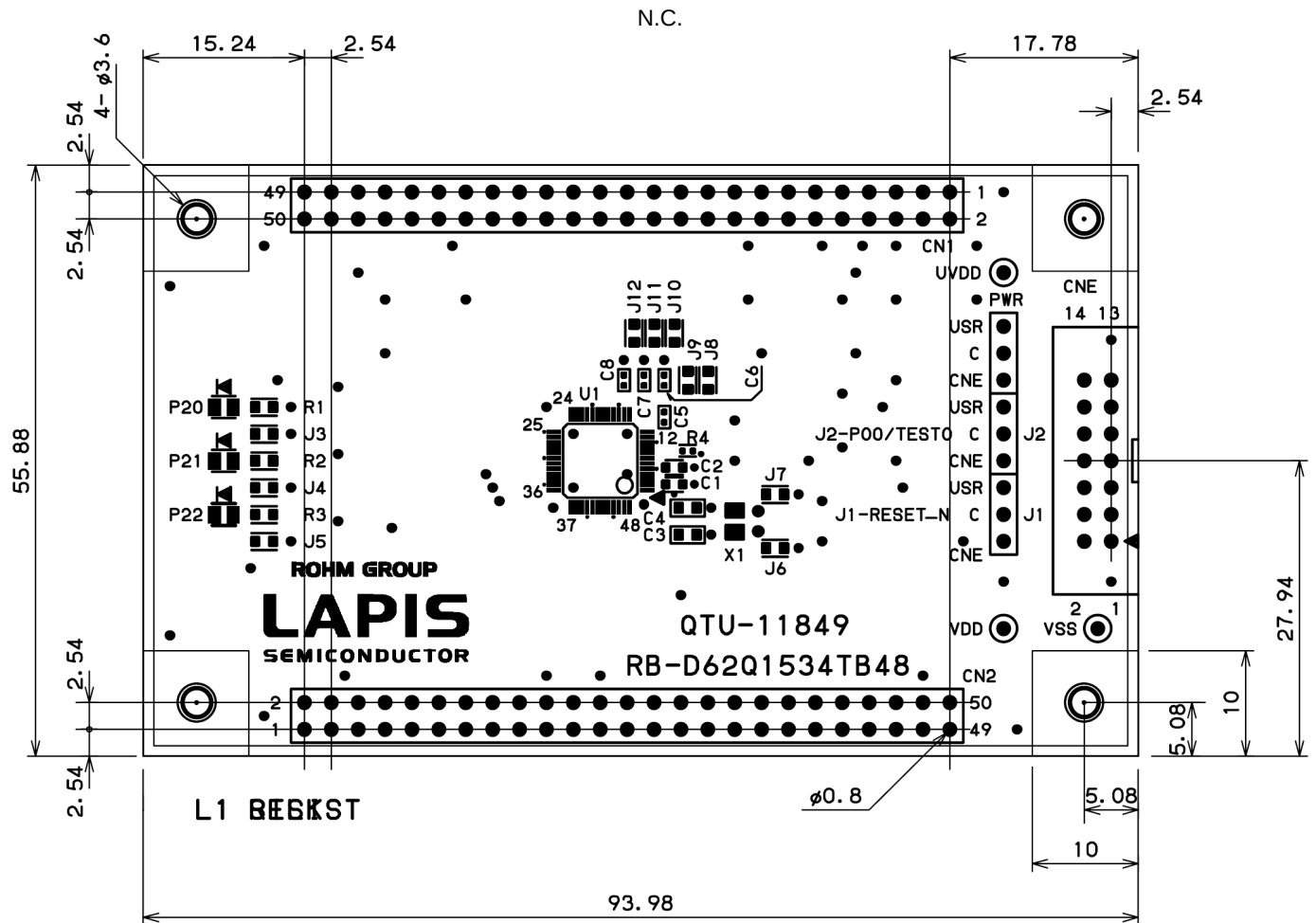
図 7 ML62Q1534 Reference Board 基板寸法図(TopView)
