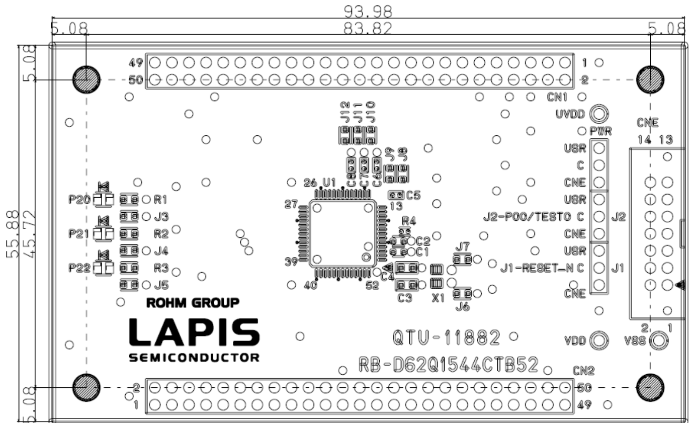
図 7 ML62Q1544C Reference Board 基板寸法図(TopView)
