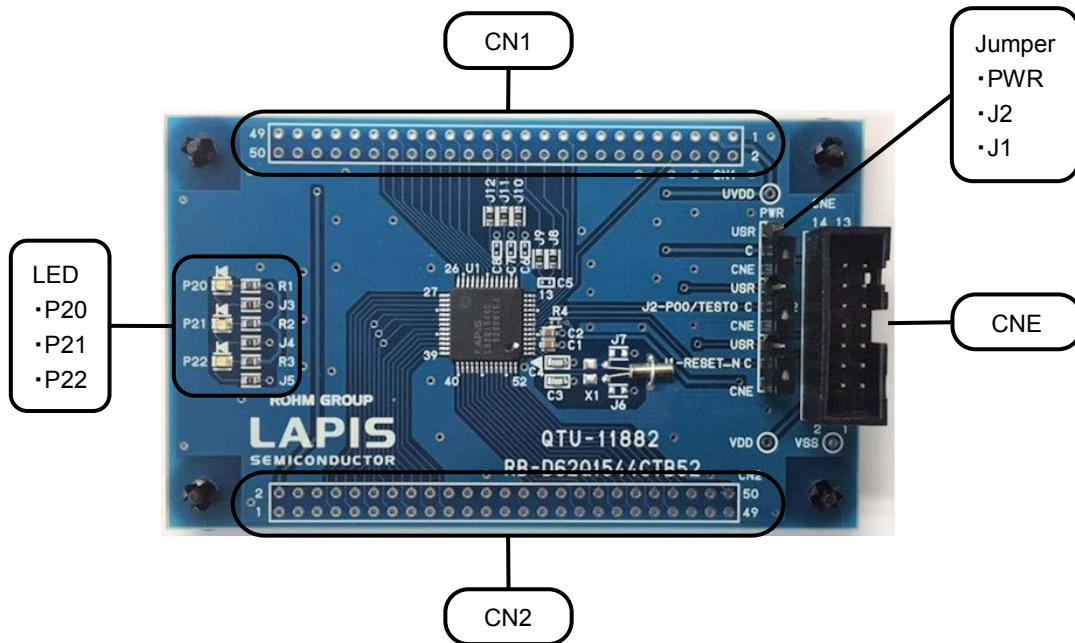
図 1 ML62Q1544C Reference Board 外観図
