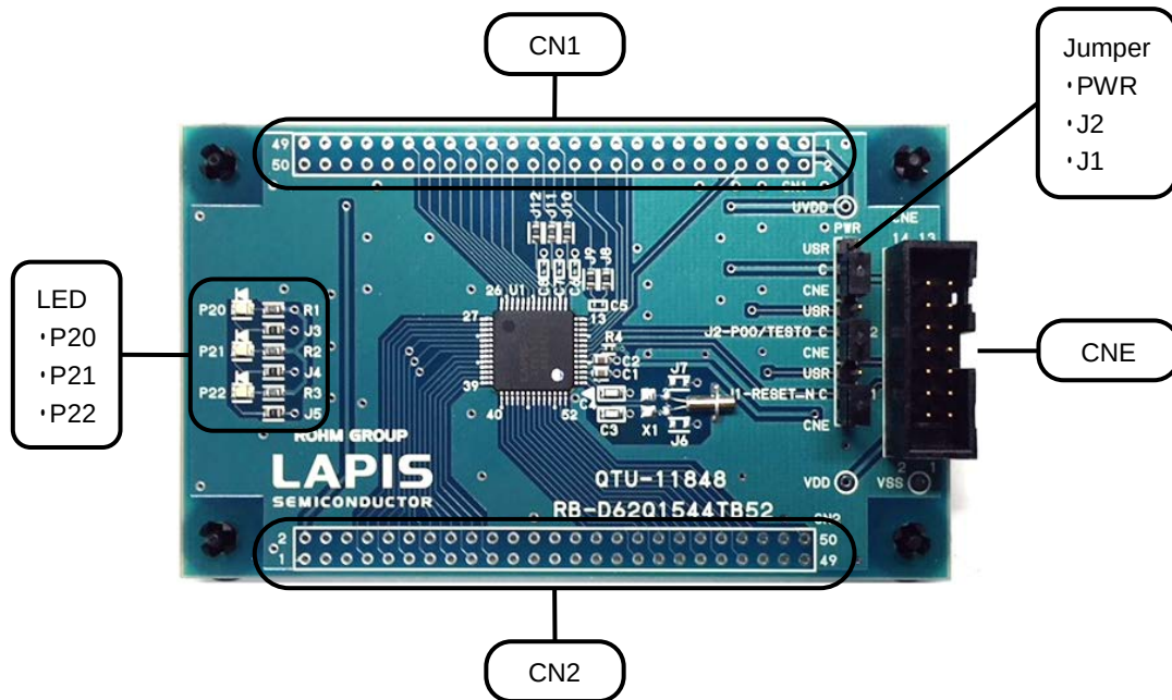
図 1 ML62Q1544 Reference Board 外観図
