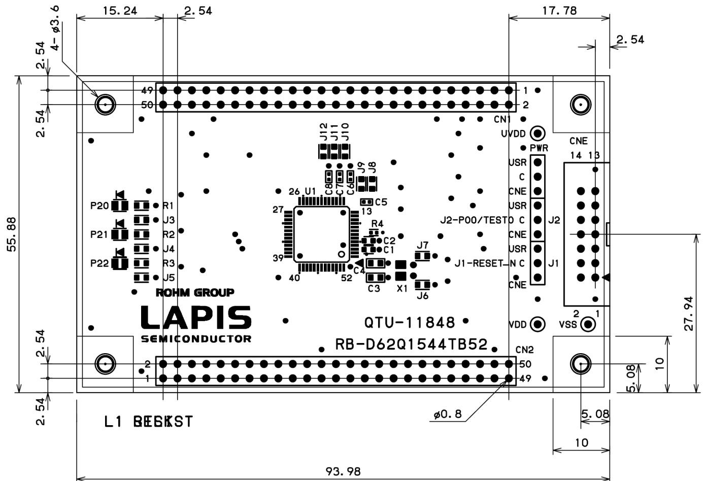
図 7 ML62Q1544 Reference Board 基板寸法図(TopView)
