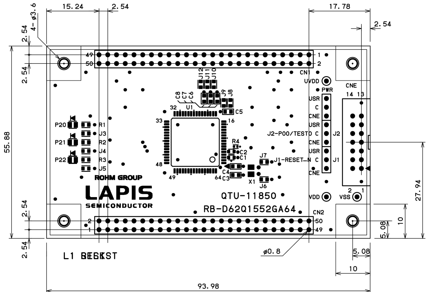
図 7 ML62Q1552 Reference Board 基板寸法図(TopView)
