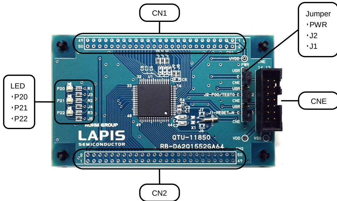
図 1 ML62Q1552 Reference Board 外観図
