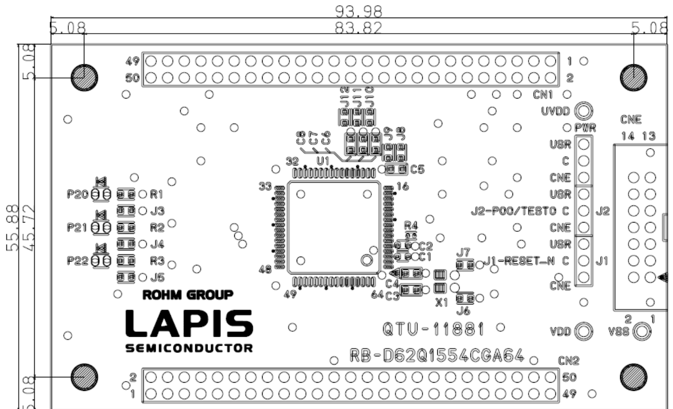
図 7 ML62Q1554C Reference Board 基板寸法図(TopView)
