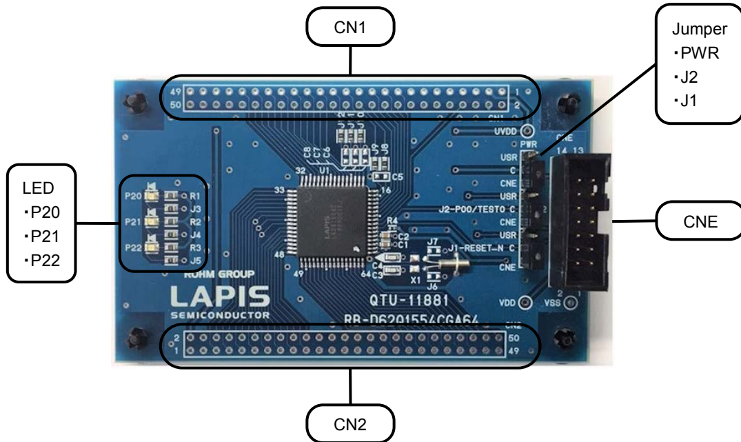
図 1 ML62Q1554C Reference Board 外観図
