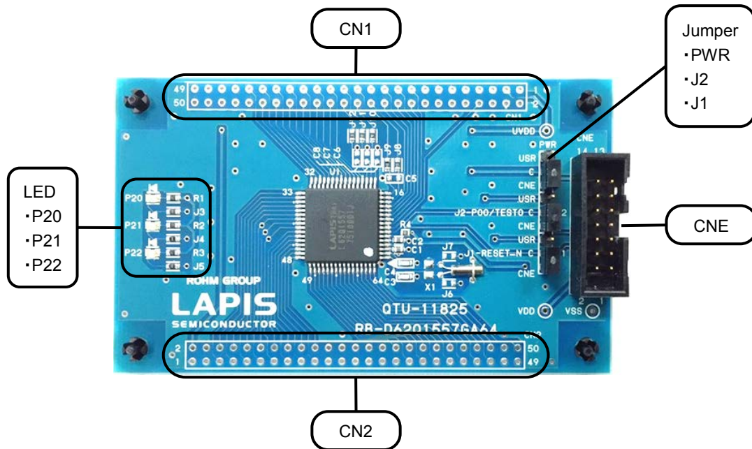
図 1 ML62Q1557 Reference Board 外観図
