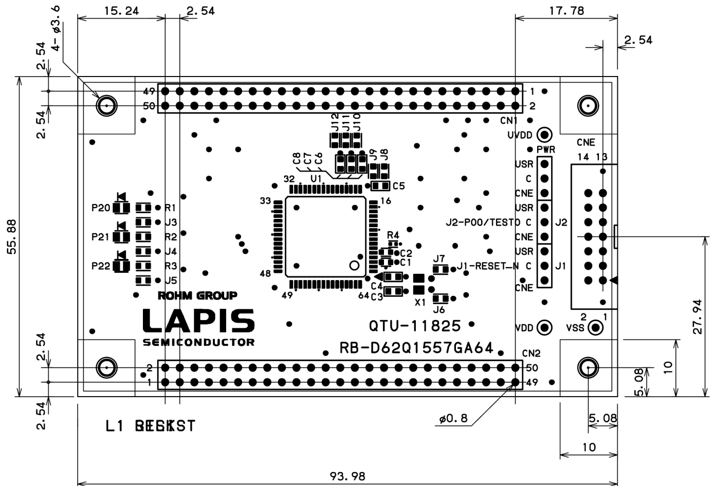
図 7 ML62Q1557 Reference Board 基板寸法図(TopView)
