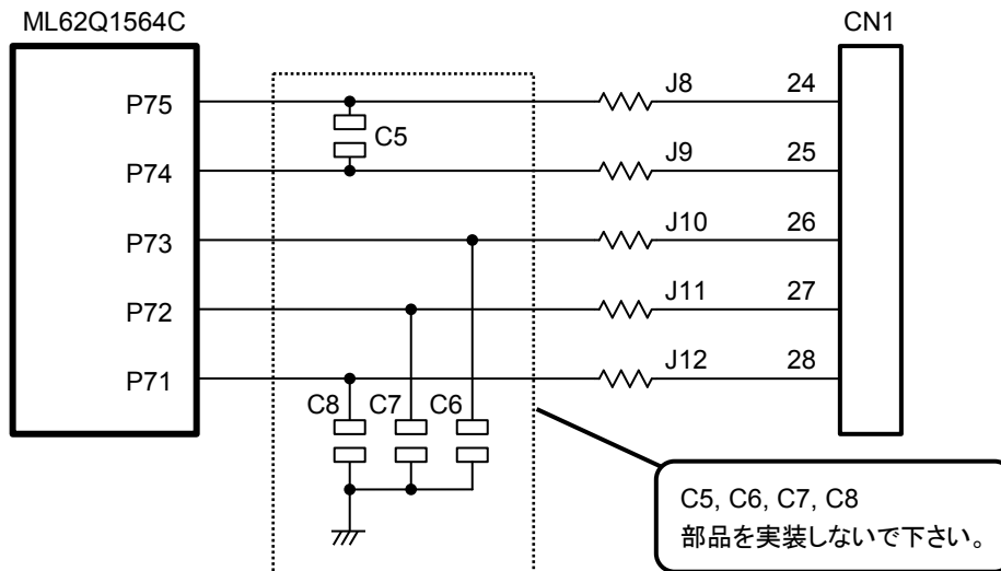
図 6 P75-P71 の回路
