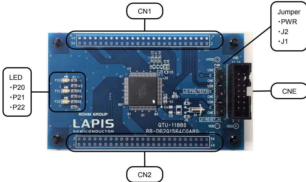
図 1 ML62Q1564C Reference Board 外観図
