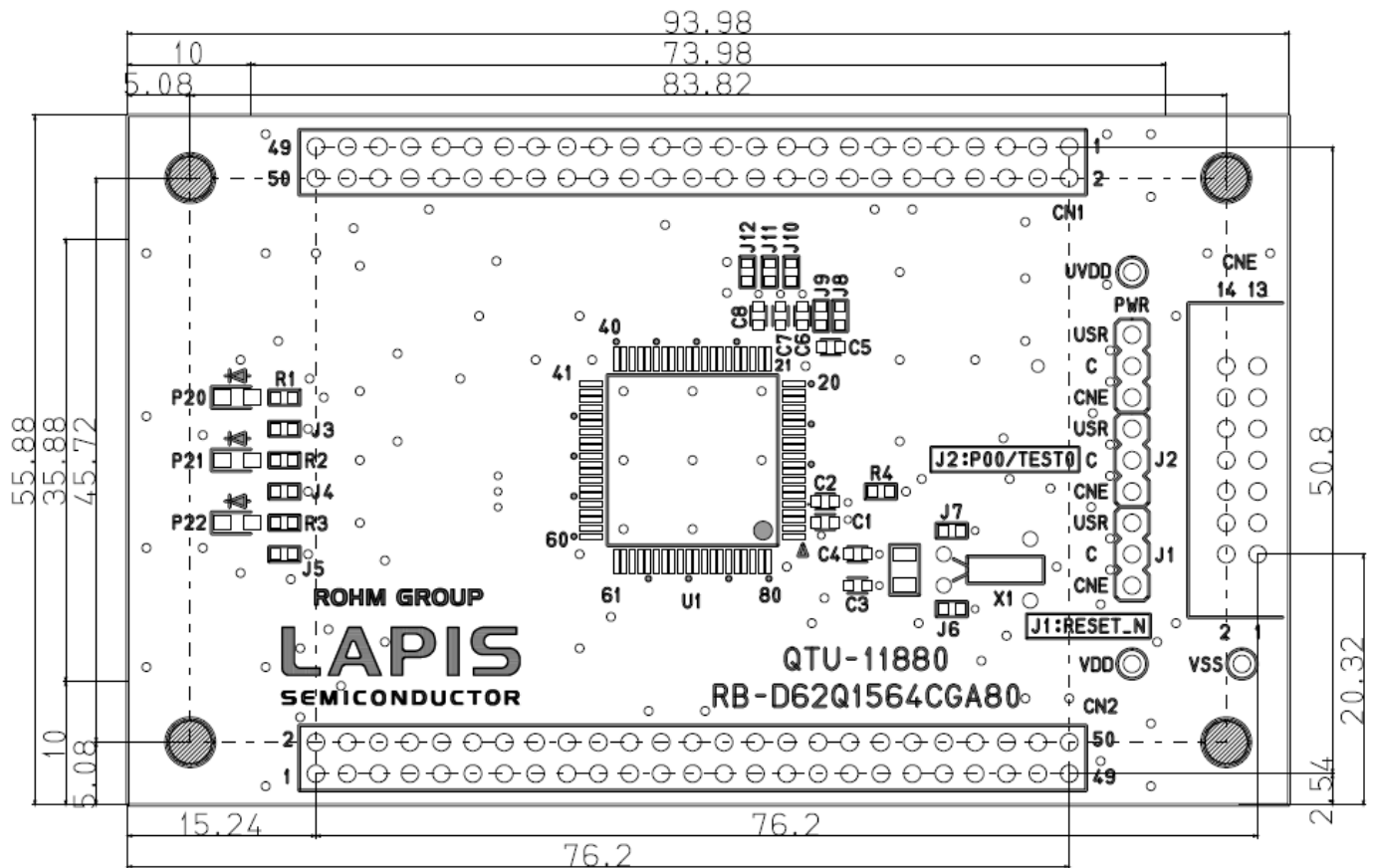
図 7 ML62Q1564C Reference Board 基板寸法図(TopView)
