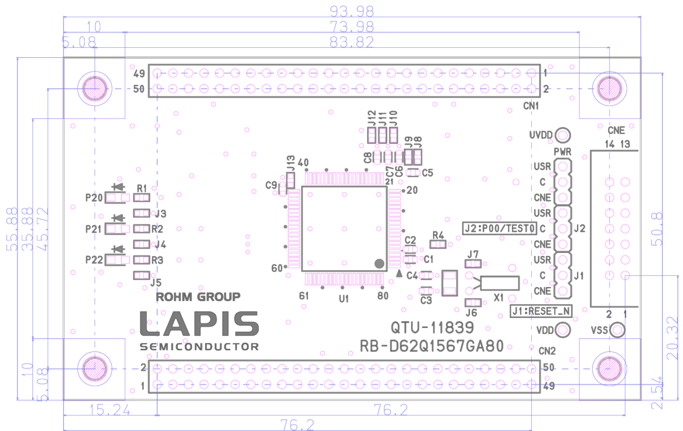
図 7 ML62Q1567 Reference Board 基板寸法図(TopView)
