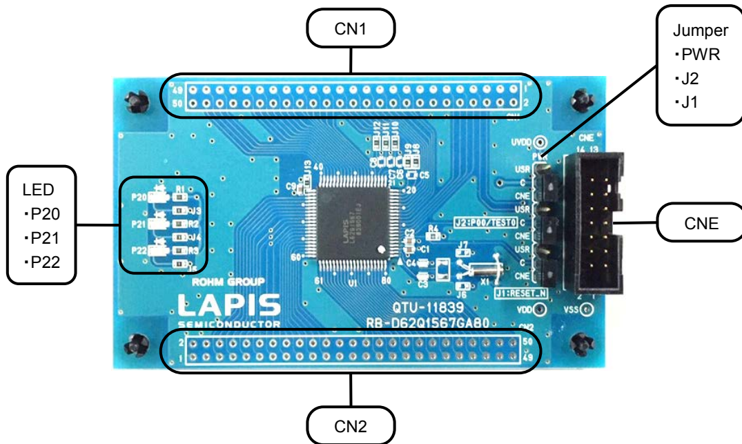
図 1 ML62Q1567 Reference Board 外観図
