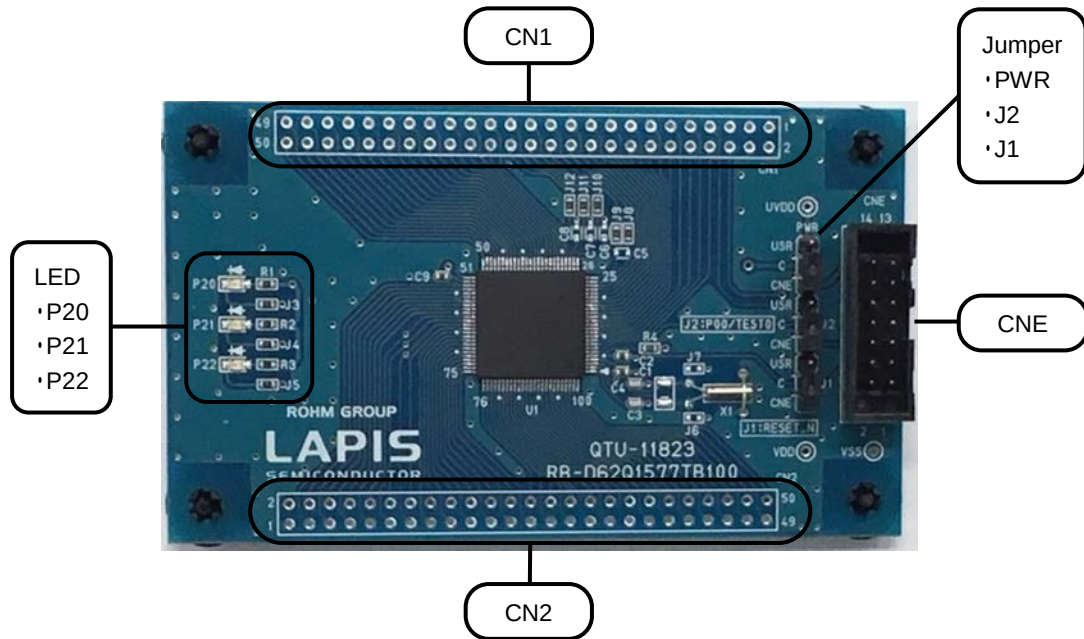
図 1 ML62Q1577 Reference Board 外観図
