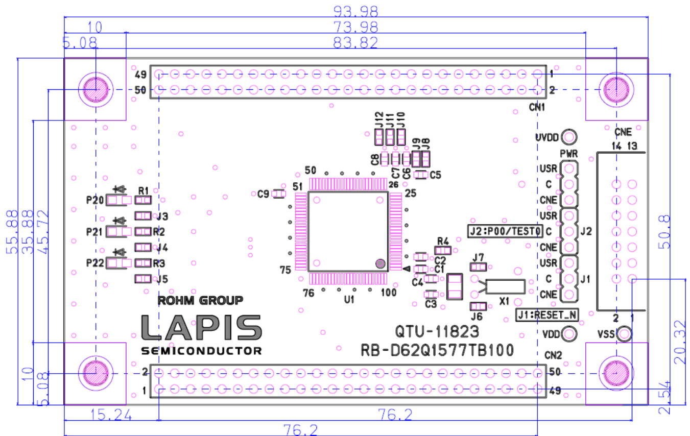
図 7 ML62Q1577 Reference Board 基板寸法図(TopView)
