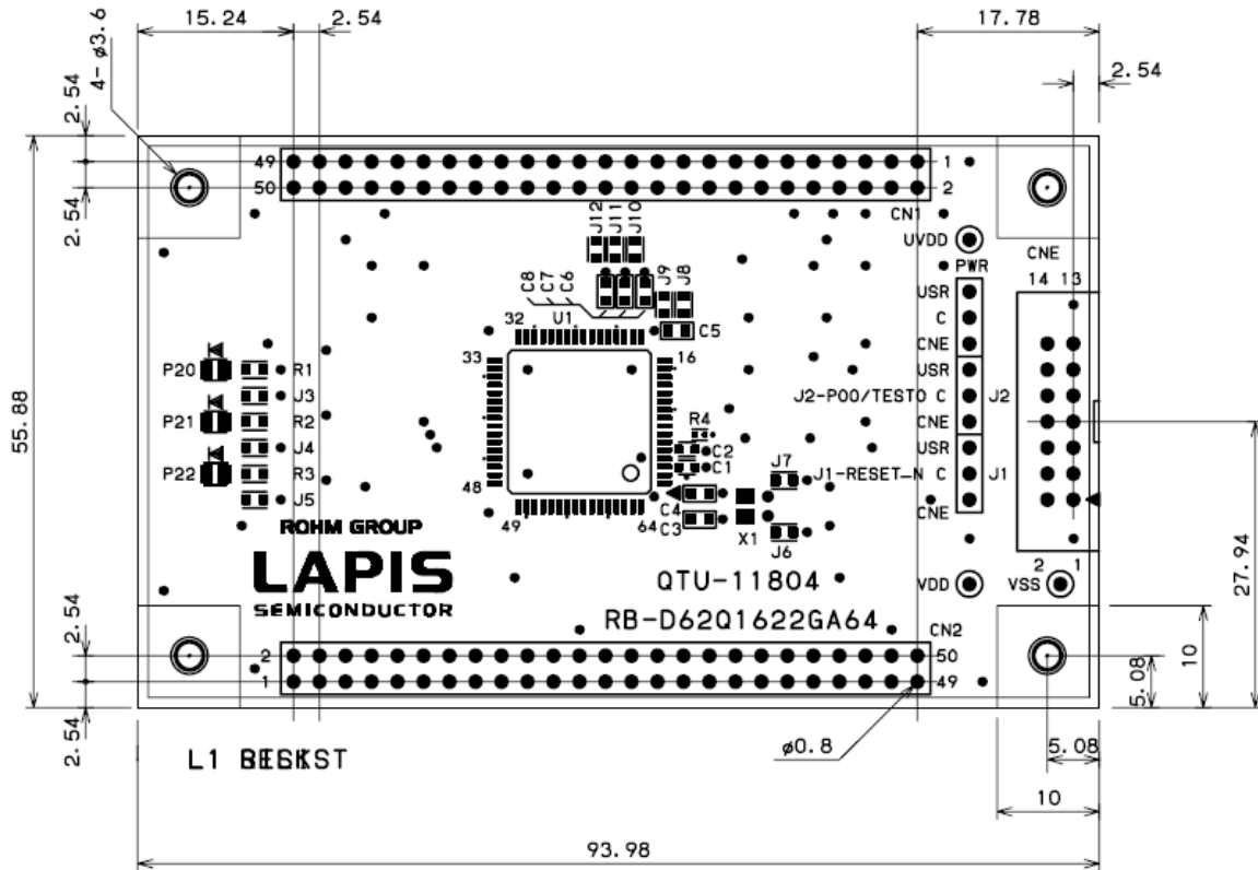
図 7. ML62Q1622 Reference Board 基板寸法図(TopView)
