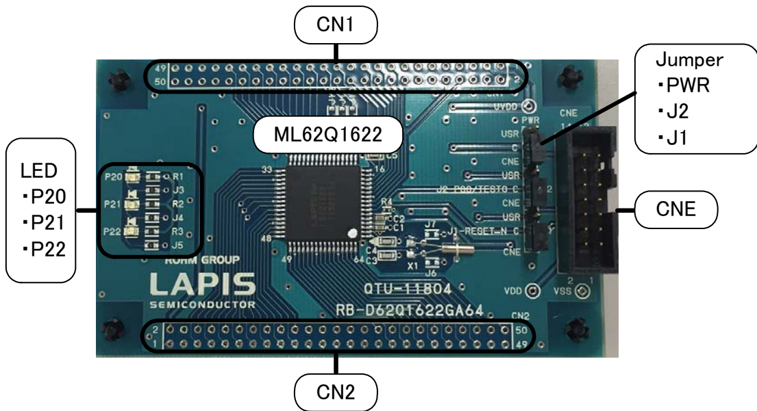
図 1. ML62Q1622 Reference Board 外観図
