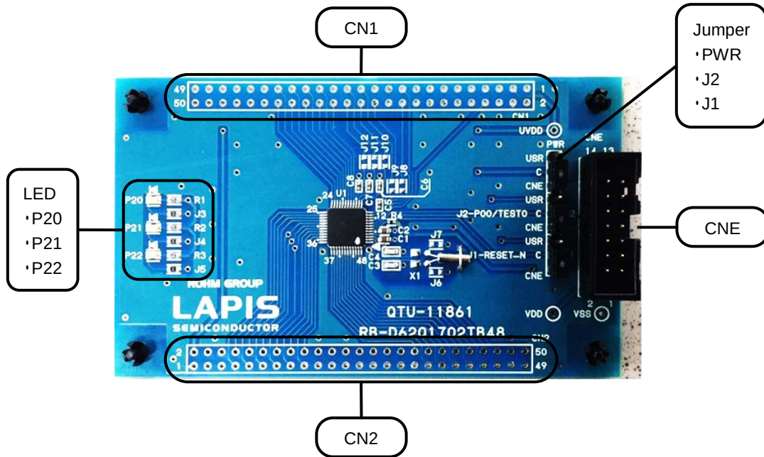
図 1 ML62Q1702 Reference Board 外観図
