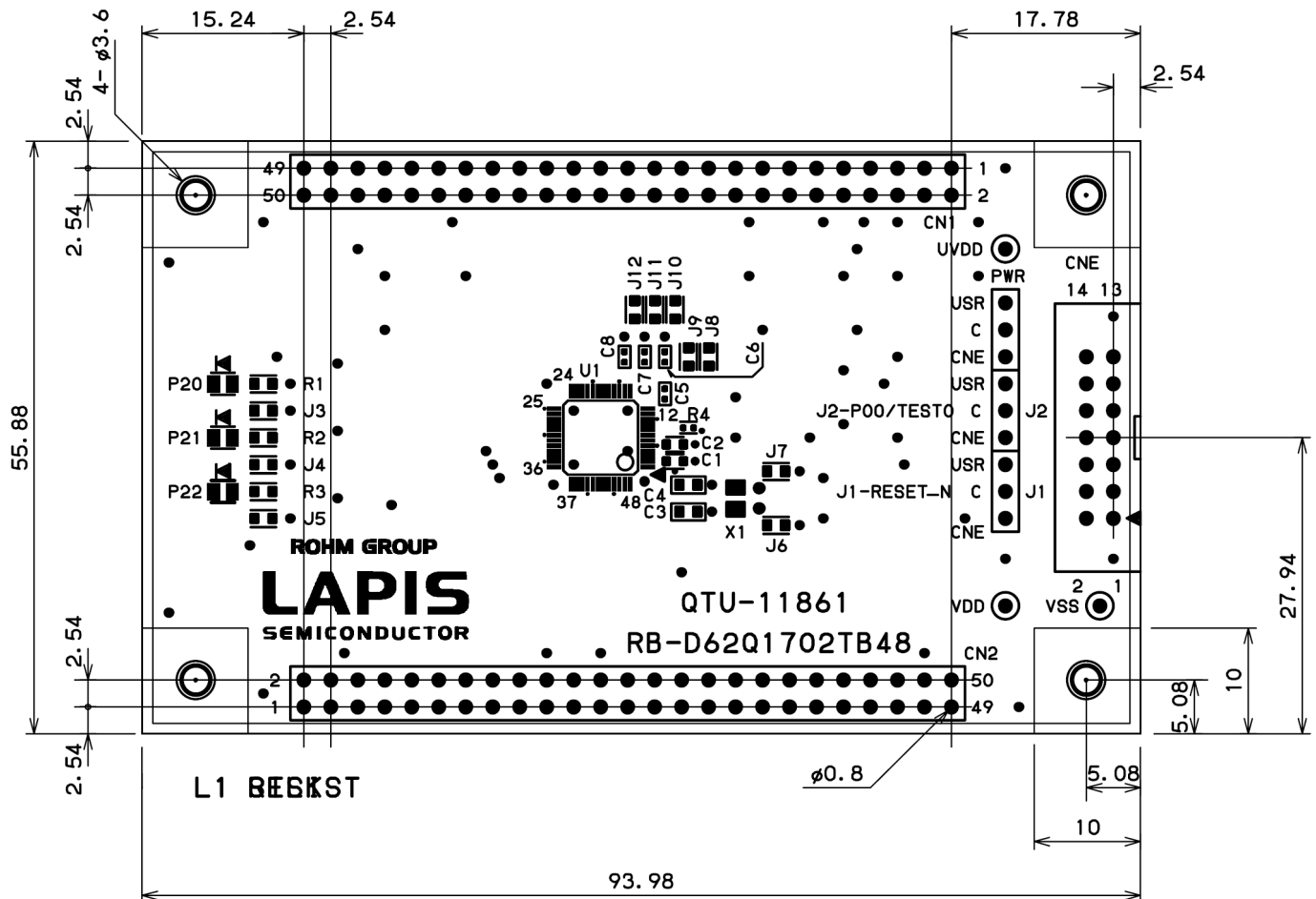
図 7 ML62Q1702 Reference Board 基板寸法図(TopView)
