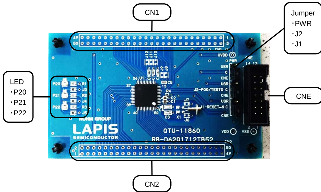
図 1 ML62Q1712 Reference Board 外観図
