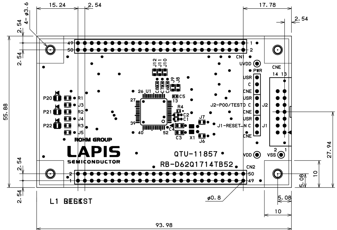
図 7 ML62Q1714 Reference Board 基板寸法図(TopView)
