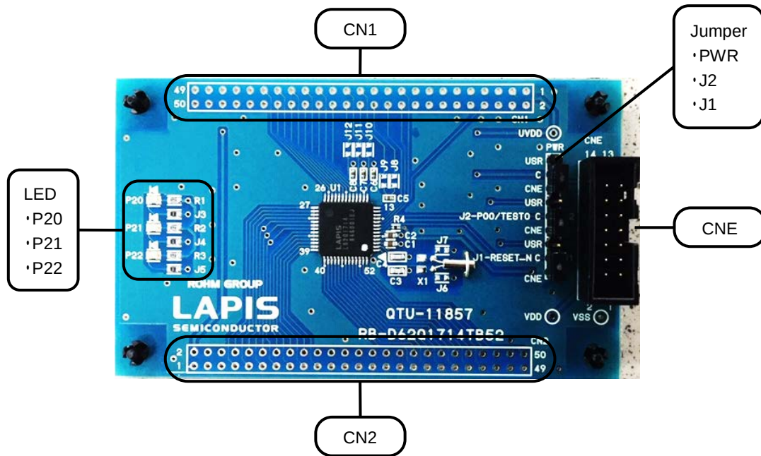
図 1 ML62Q1714 Reference Board 外観図
