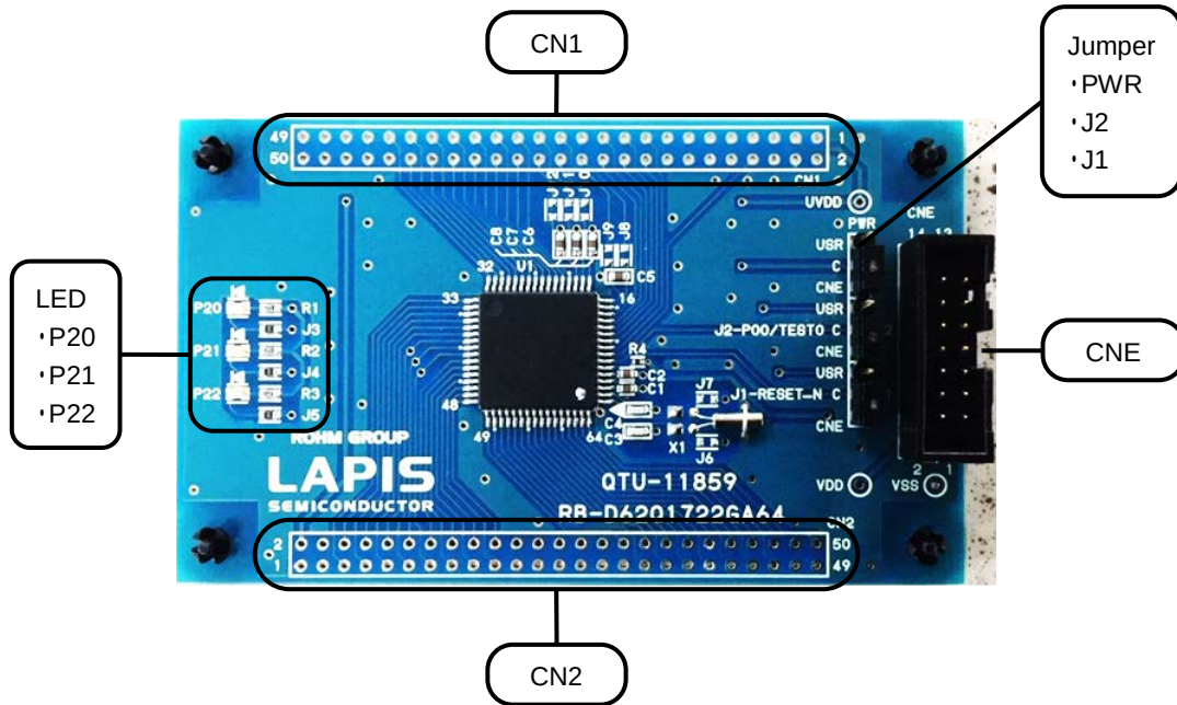
図 1 ML62Q1722 Reference Board 外観図
