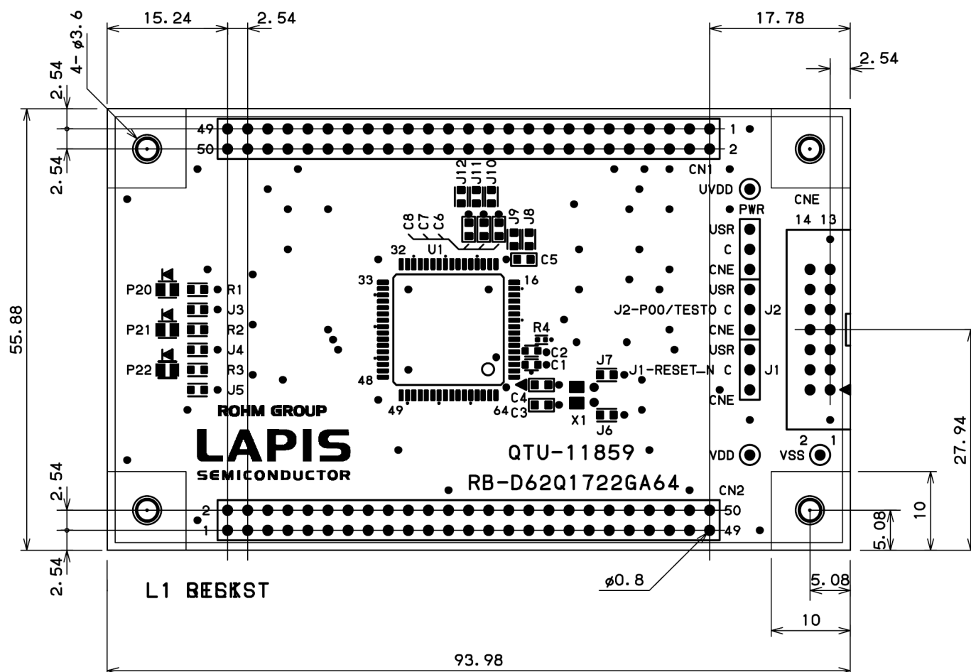
图 7 ML62Q1722 Reference Board 基板寸法图(TopView)
