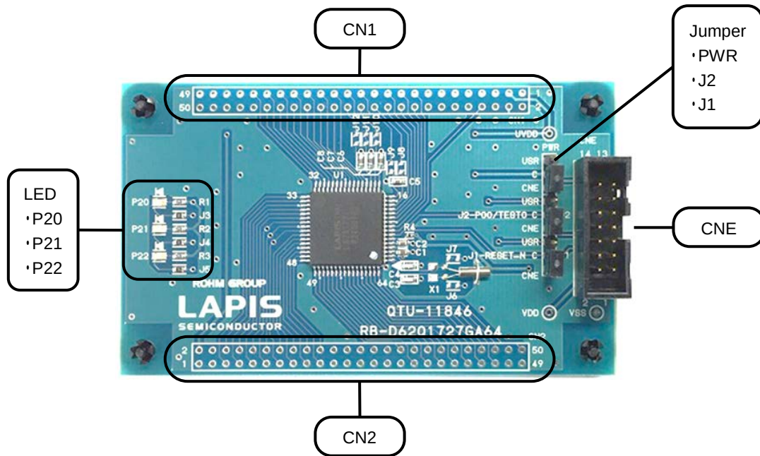
図 1 ML62Q1727 Reference Board 外観図
