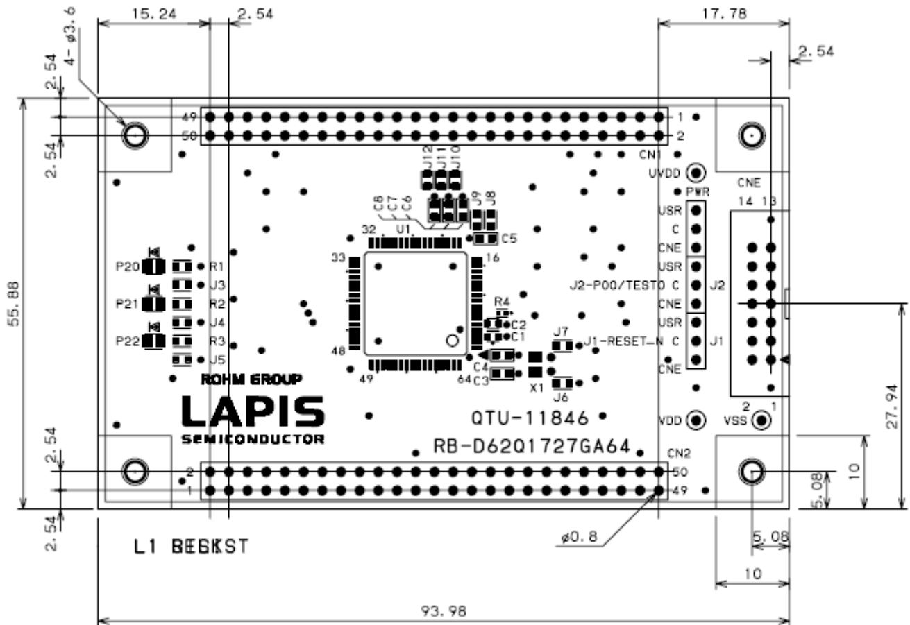
図 7 ML62Q1727 Reference Board 基板寸法図(TopView)
