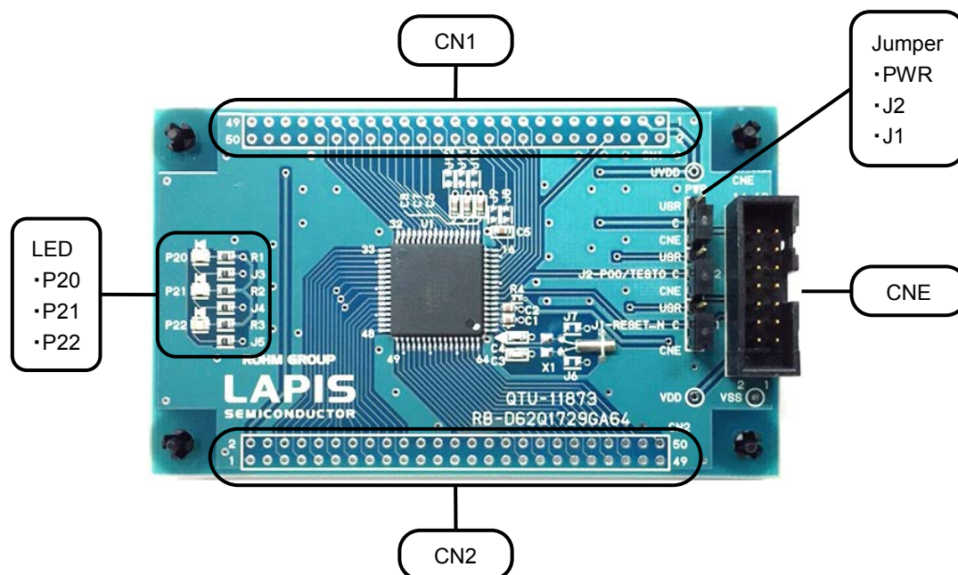
図 1 ML62Q1729 Reference Board 外観図
