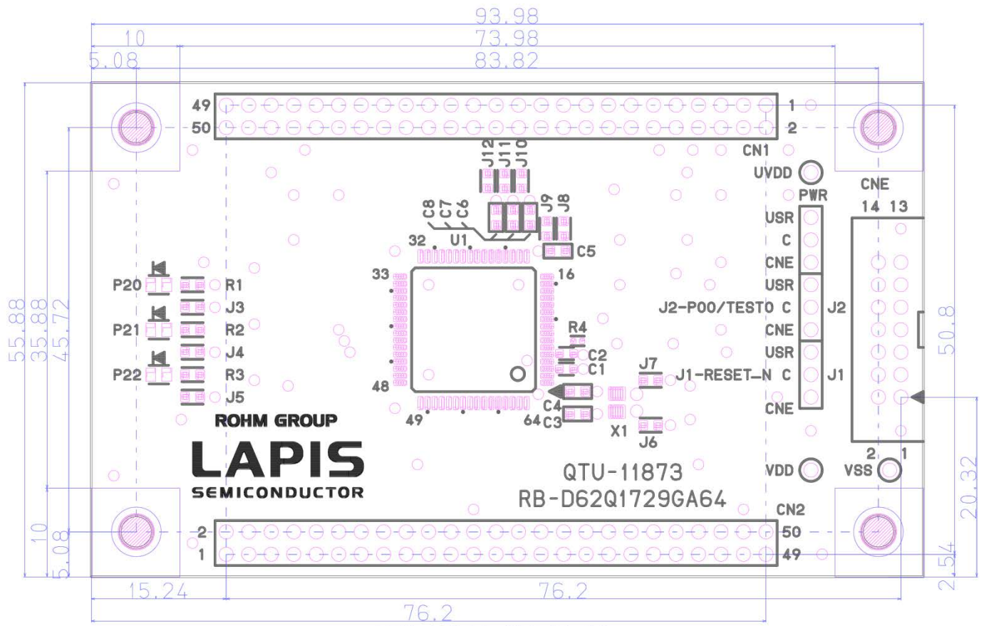
図 7 ML62Q1729 Reference Board 基板寸法図(TopView)
