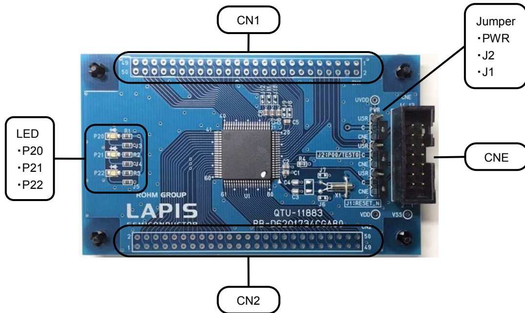
図 1 ML62Q1734C Reference Board 外観図
