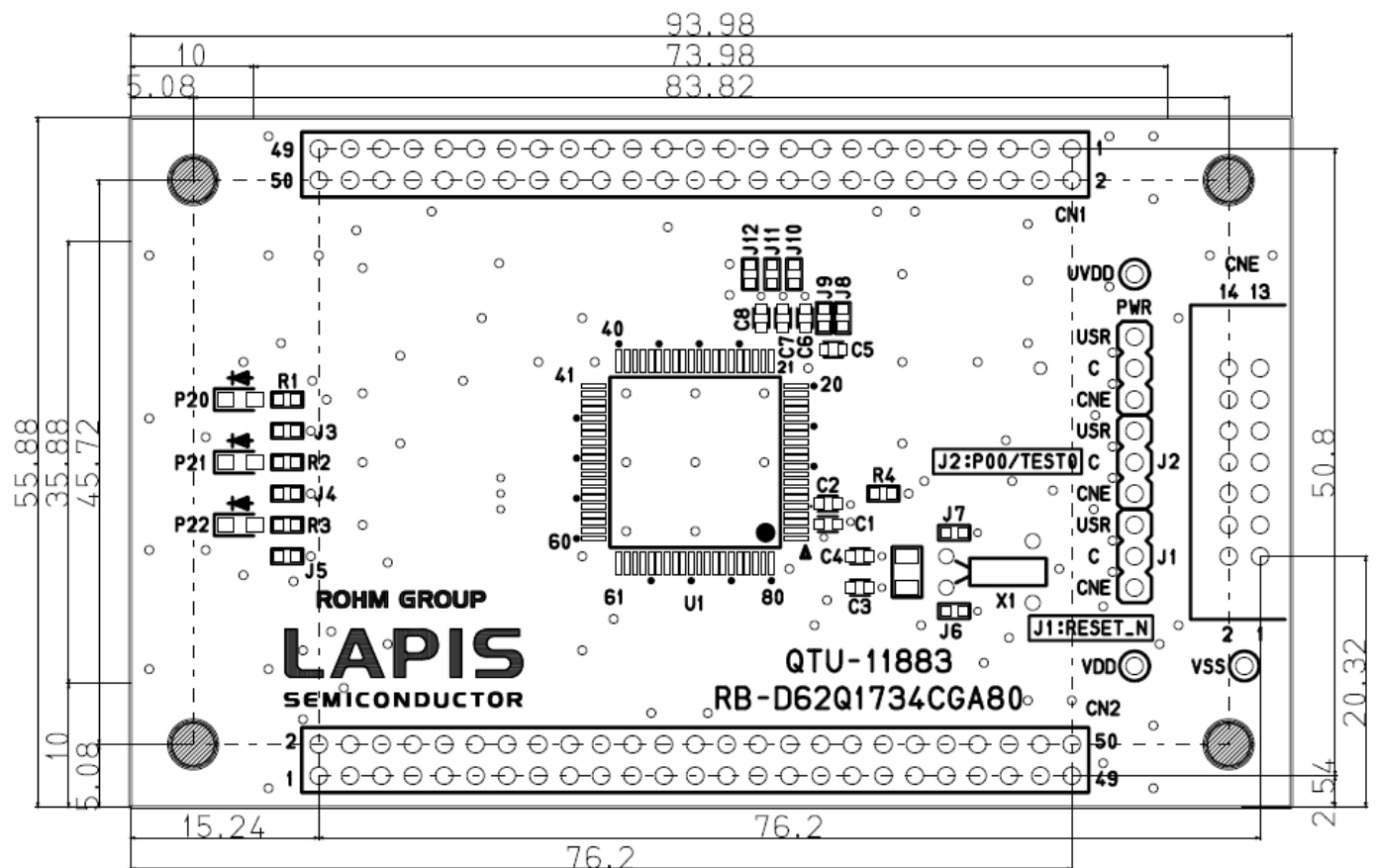
図 7 ML62Q1734C Reference Board 基板寸法図(TopView)
