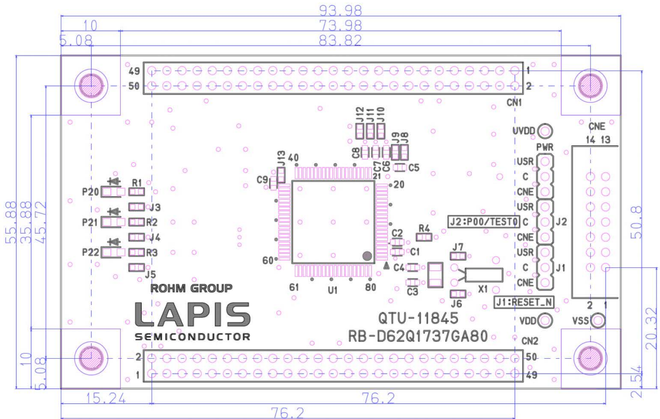
図 7 ML62Q1737 Reference Board 基板寸法図(TopView)
