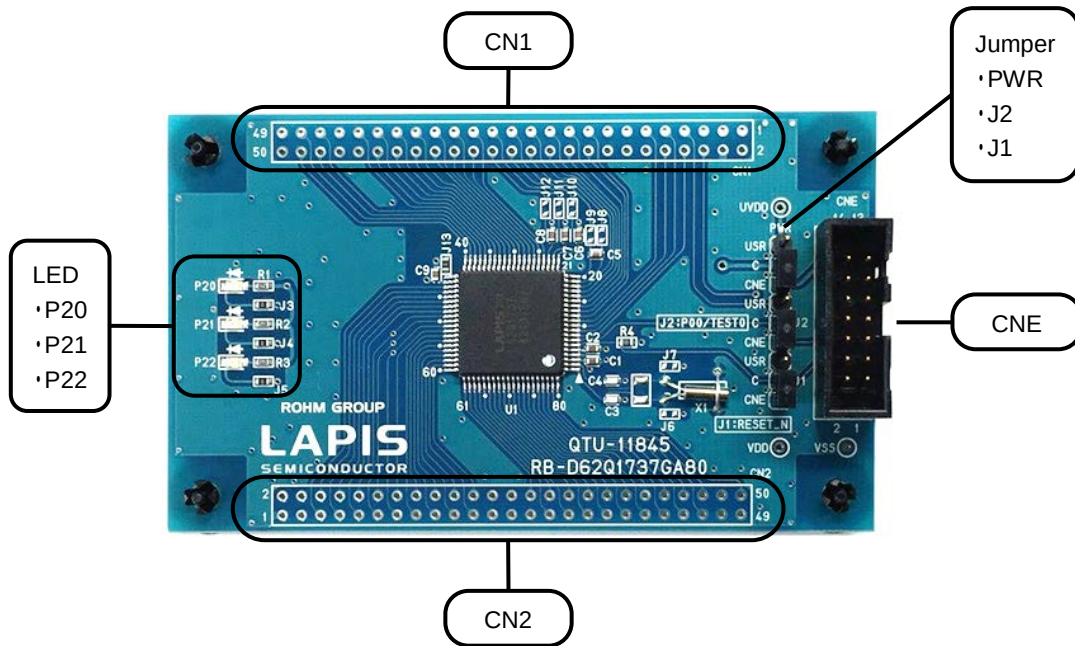
図 1 ML62Q1737 Reference Board 外観図
