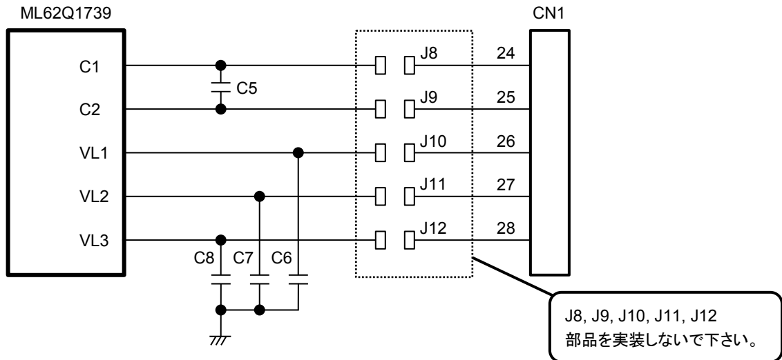
図 6 C1, C2, VL1, VL2, VL3 の回路
