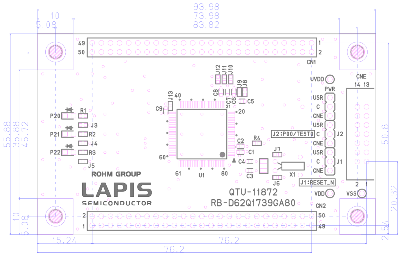
図 7 ML62Q1739 Reference Board 基板寸法図(TopView)
