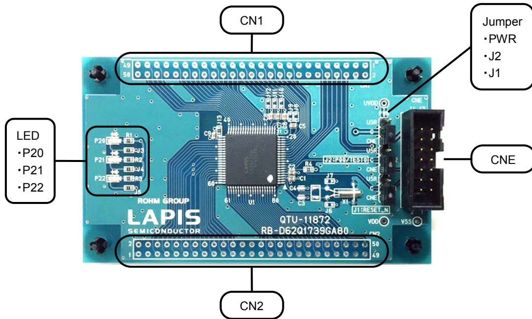
図 1 ML62Q1739 Reference Board 外観図
