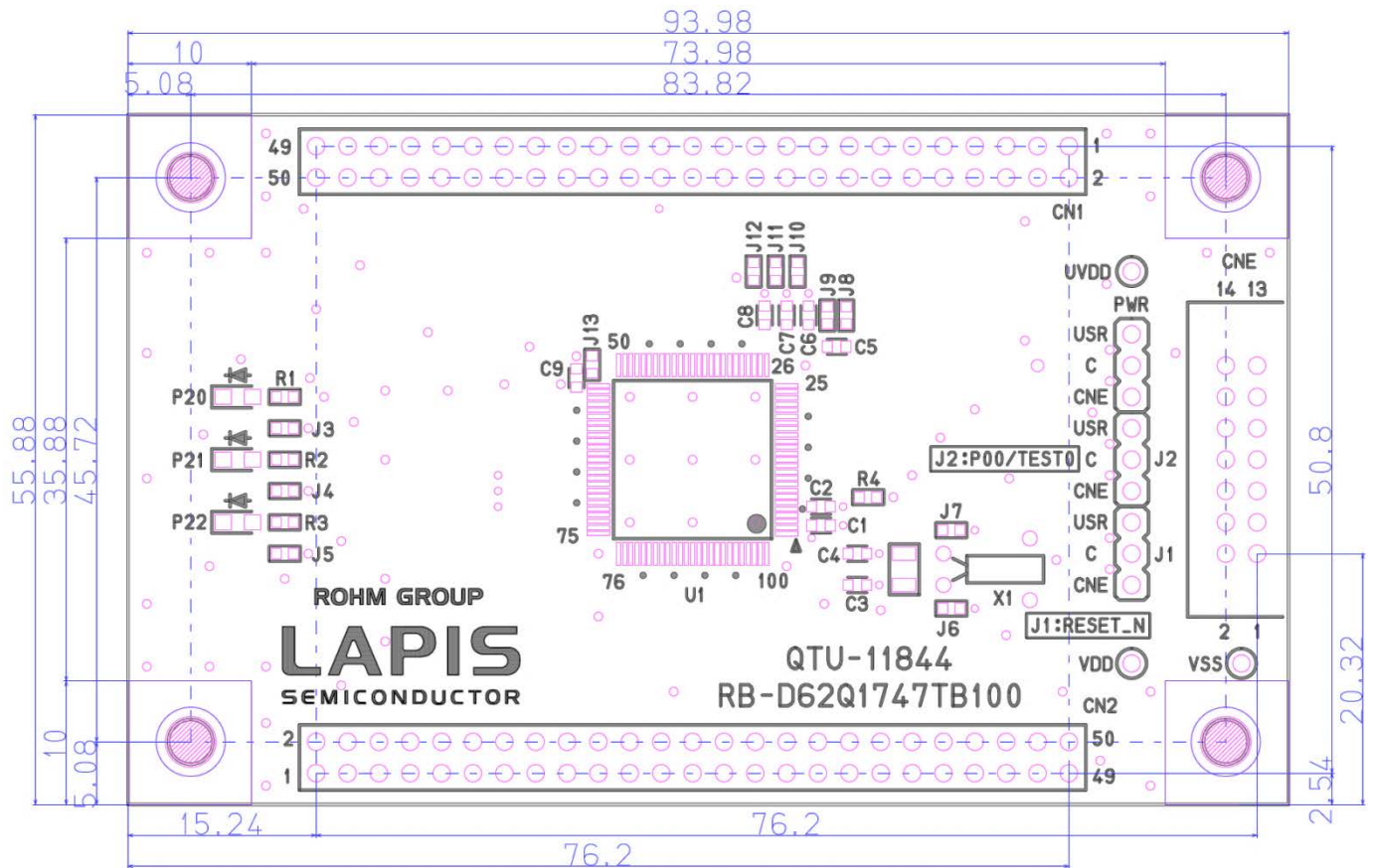
図 7 ML62Q1747 Reference Board 基板寸法図(TopView)
