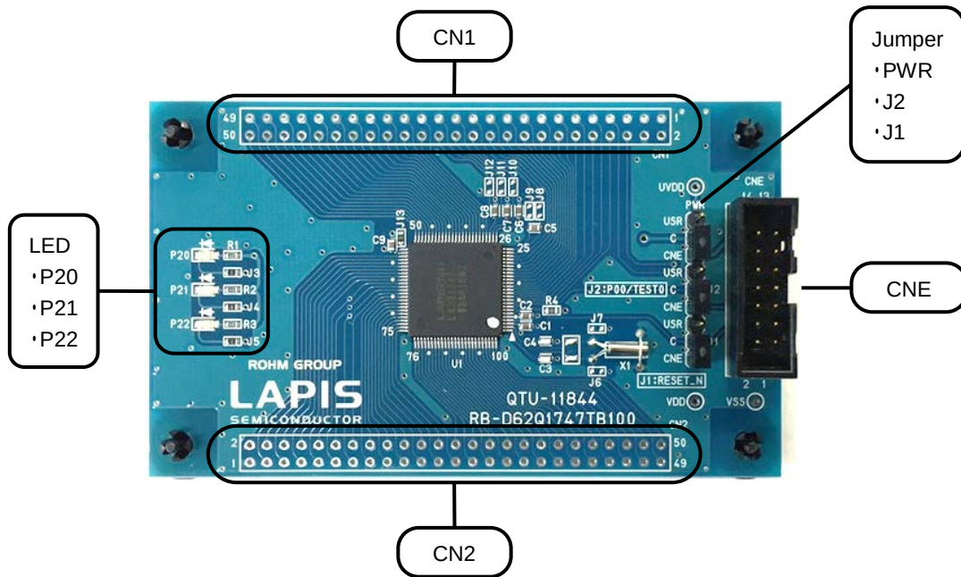
図 1 ML62Q1747 Reference Board 外観図
