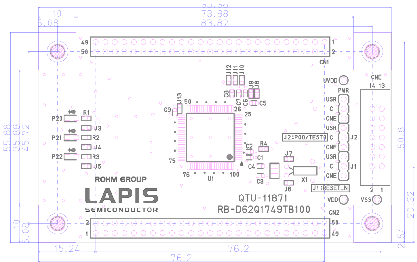
図 7 ML62Q1749 Reference Board 基板寸法図(TopView)
