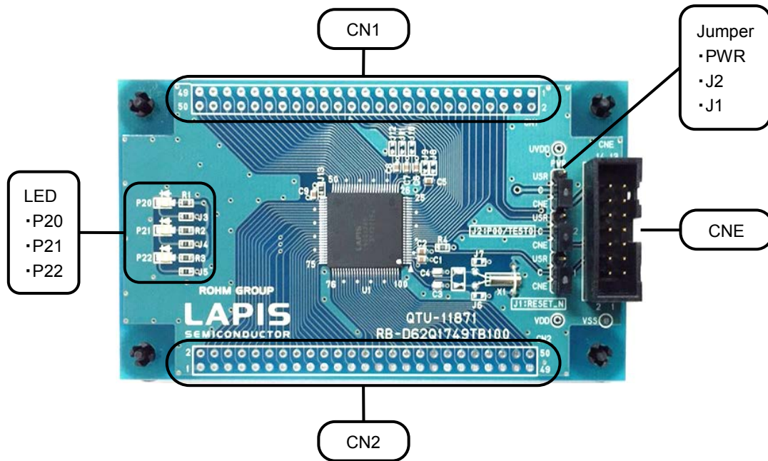
図 1 ML62Q1749 Reference Board 外観図
