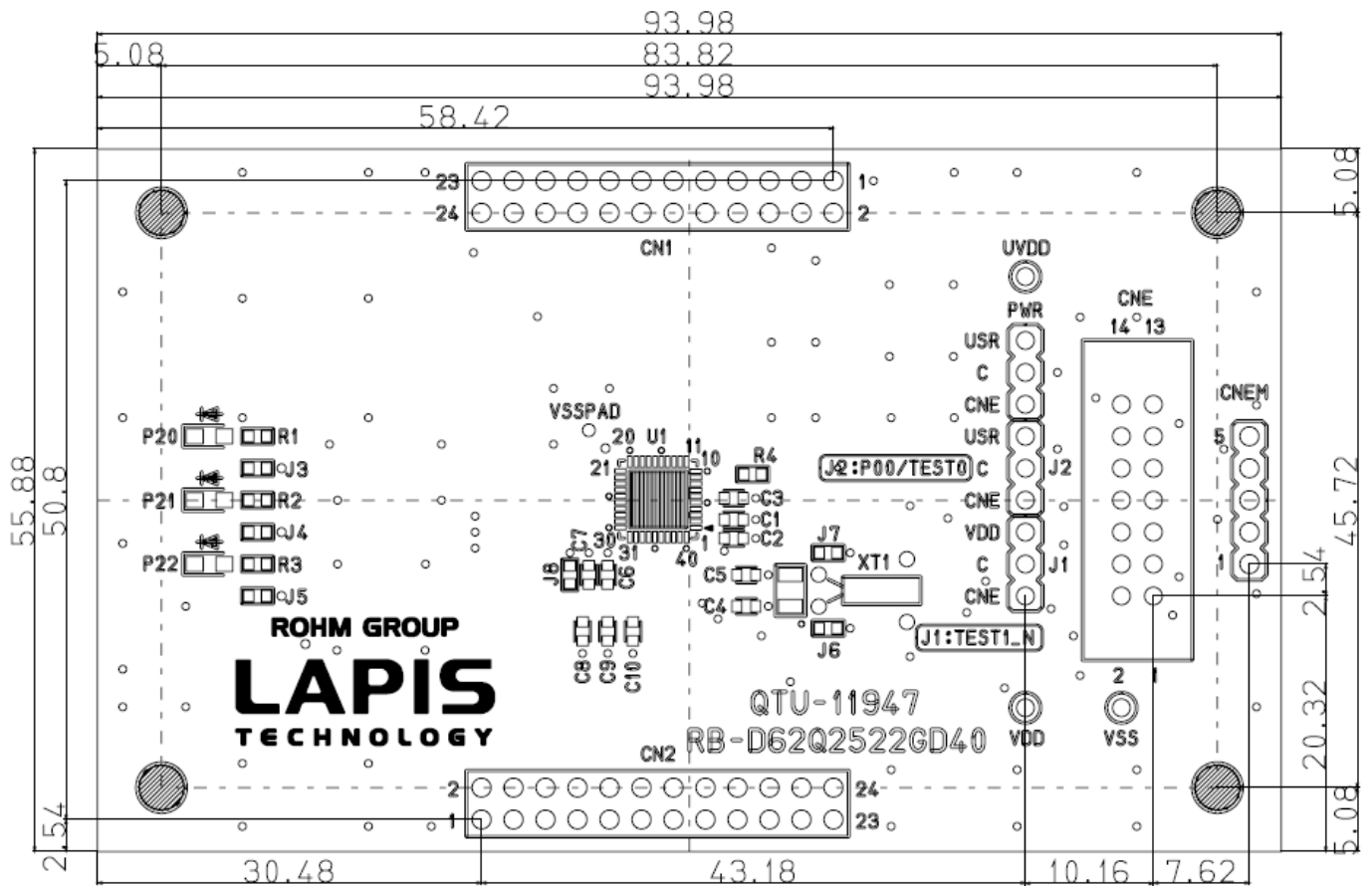
図 7 RB-D62Q2522GD40 基板寸法図 (Top View)
