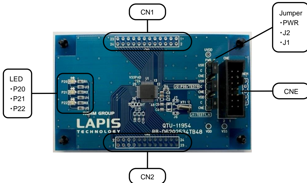
図 1 外観図
