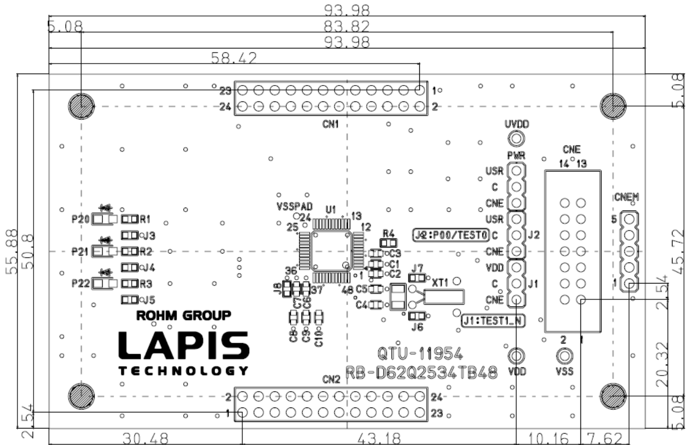
図 7 RB-D62Q2534TB48 基板寸法図 (Top View)
