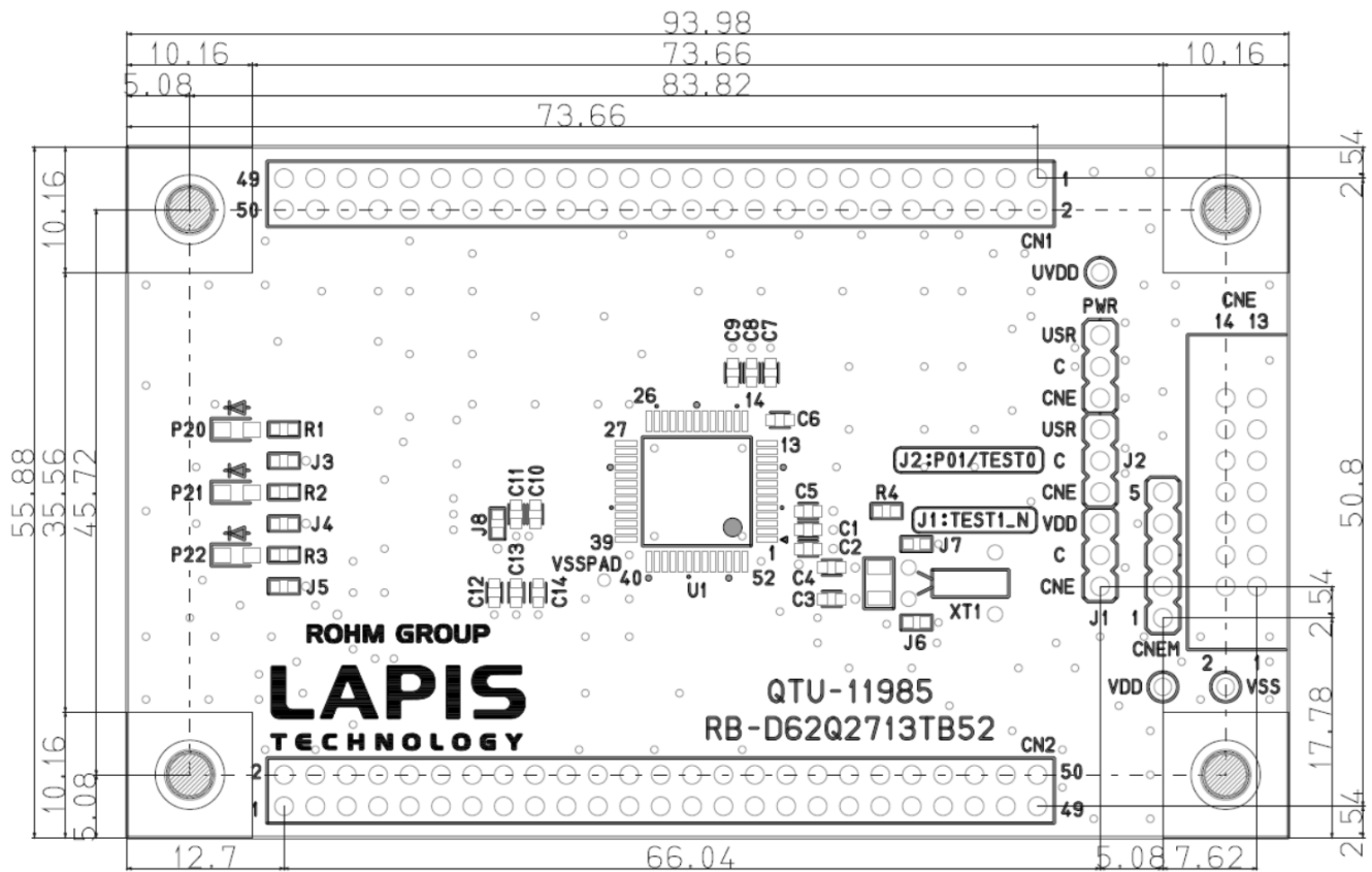
図 8 RB-D62Q2713TB52 基板寸法図 (Top View)
