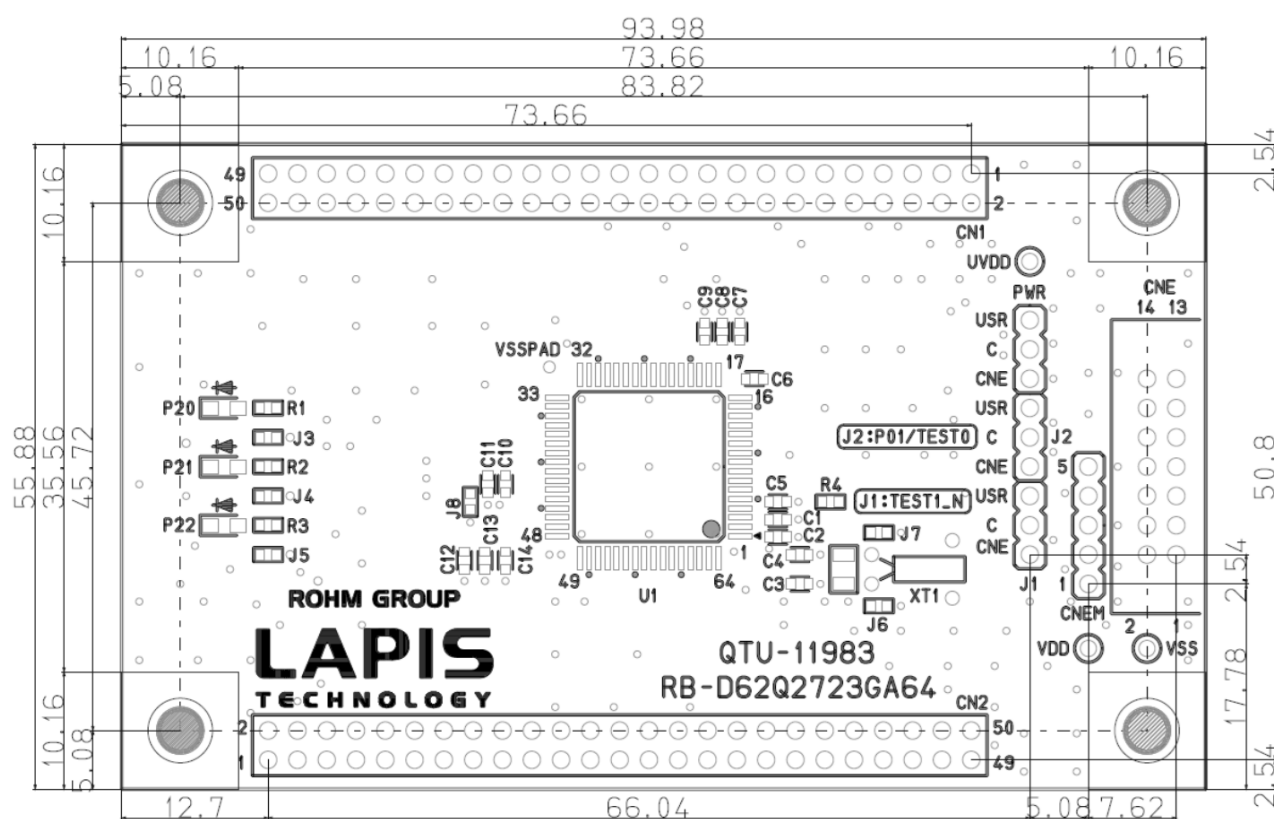
図 7 RB-D62Q2723GA64 基板寸法図 (Top View)
