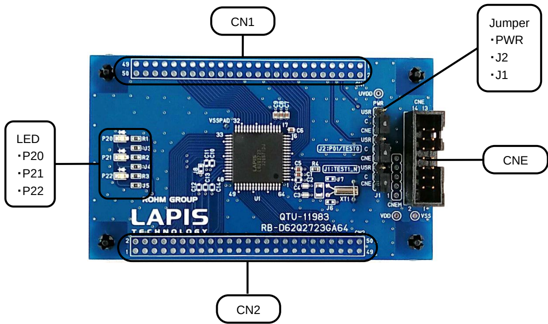
図 1 外観図
