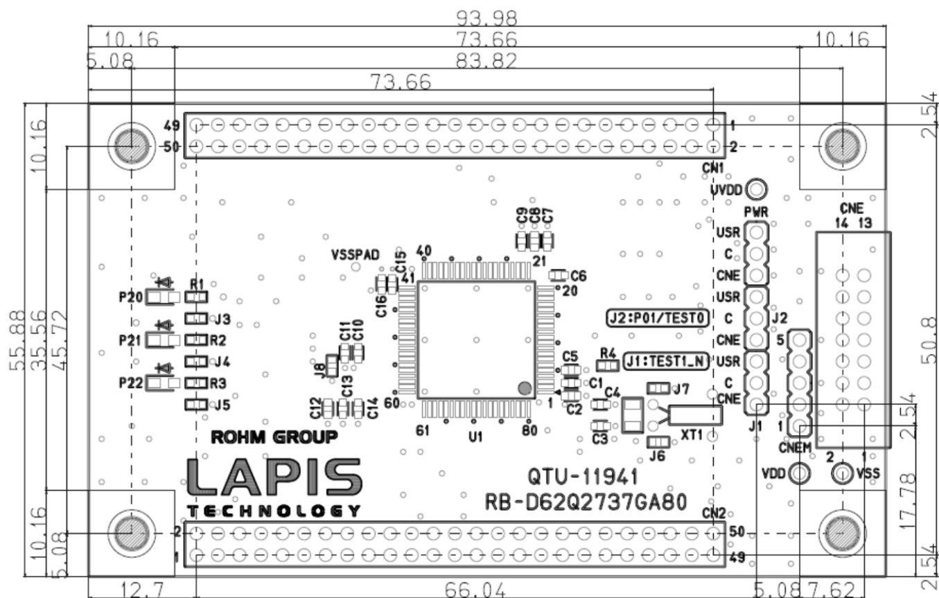
図 7 RB-D62Q2737GA80 基板寸法図 (Top View)
