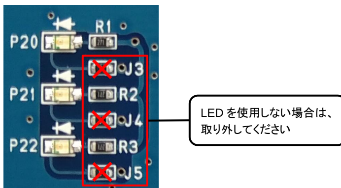
図 4 LED 廻りの加工例
