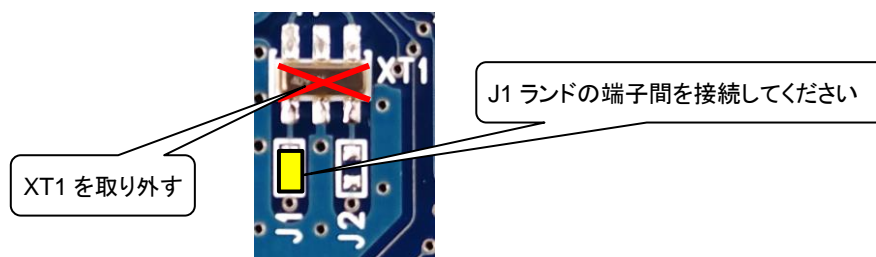
図 5 J1 ランド
