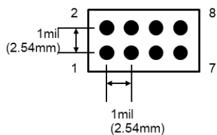
図 7 CN3 スルーホール形状
