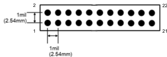
図 6 CN2 スルーホール形状
