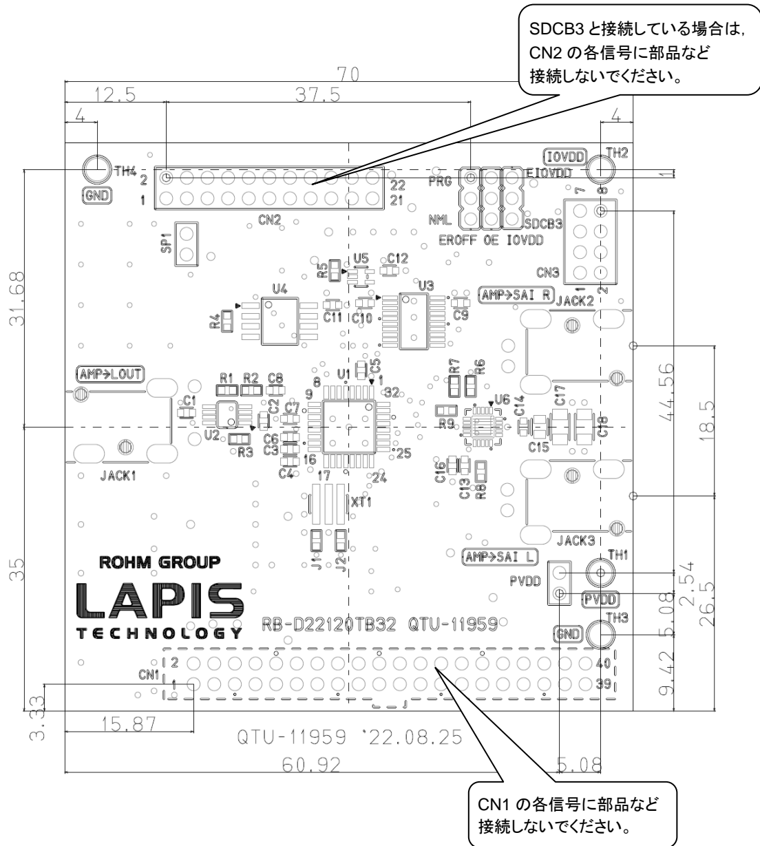
図 8 配置図
