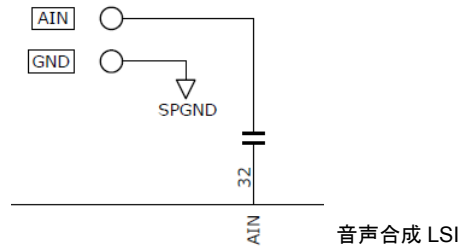
図 2 AIN スルーホール
