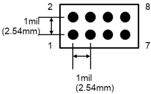
図 9 CN3 スルーホール形状
