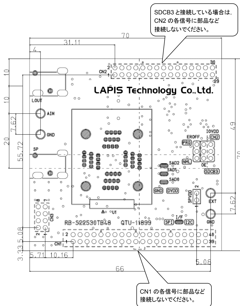
図 10 配置図
