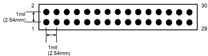
図 8 CN2 スルーホール形状
