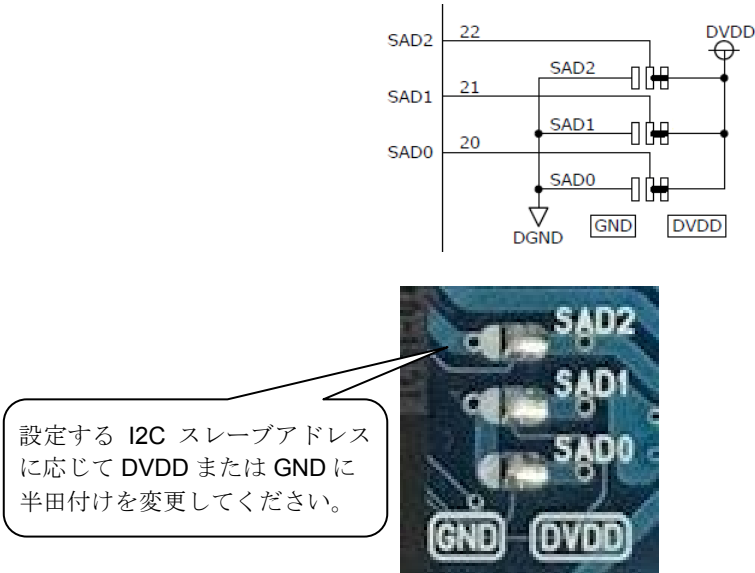
図 4 SAD2-0 ランド
