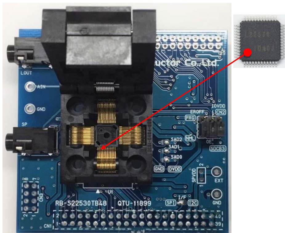
図 1 外観
