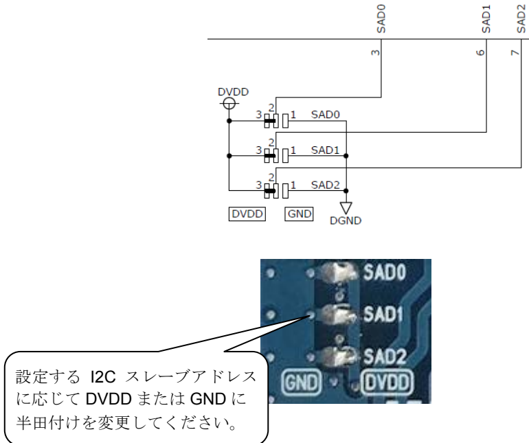
図 4 SAD2-0 ランド
