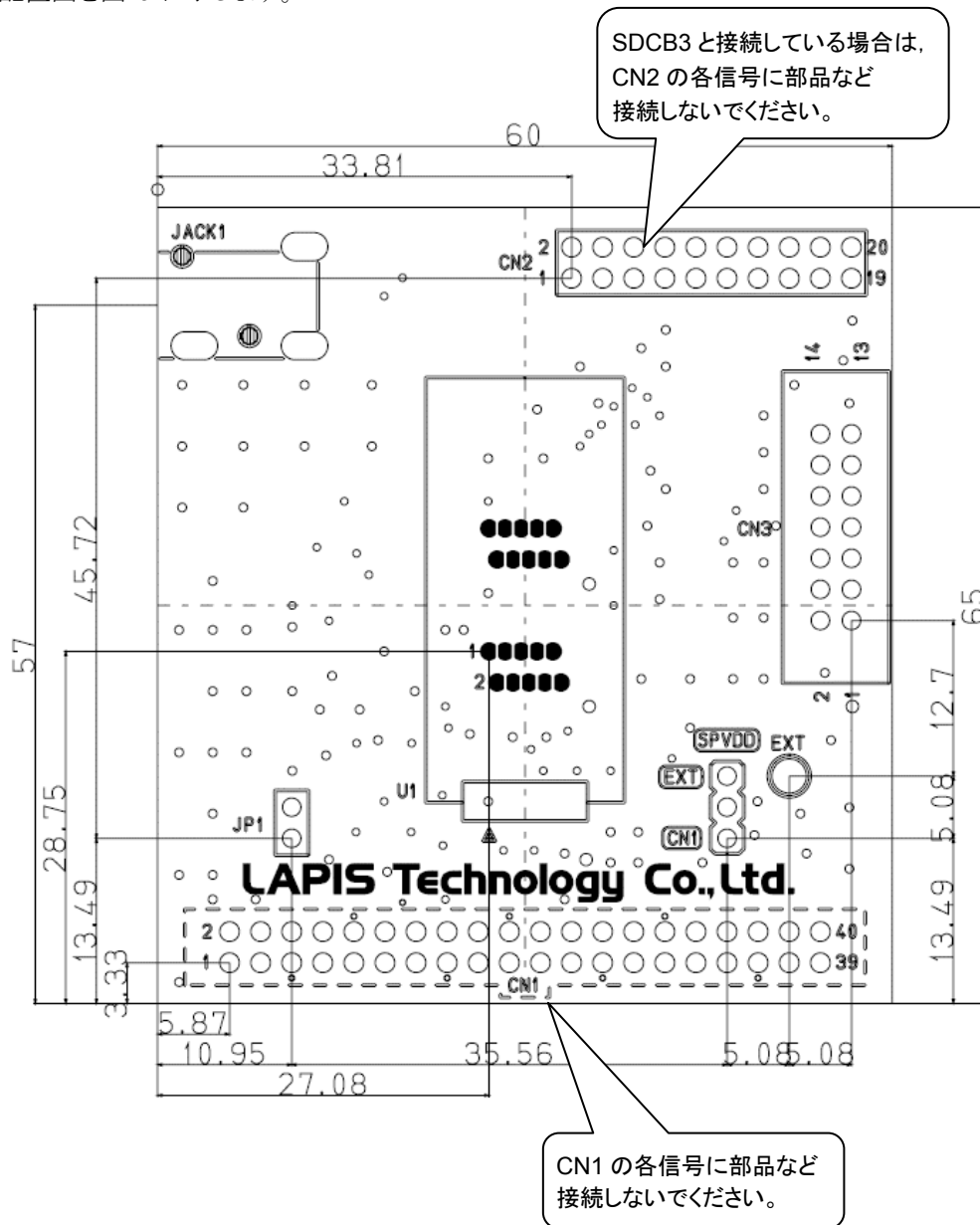
図 5 配置図
