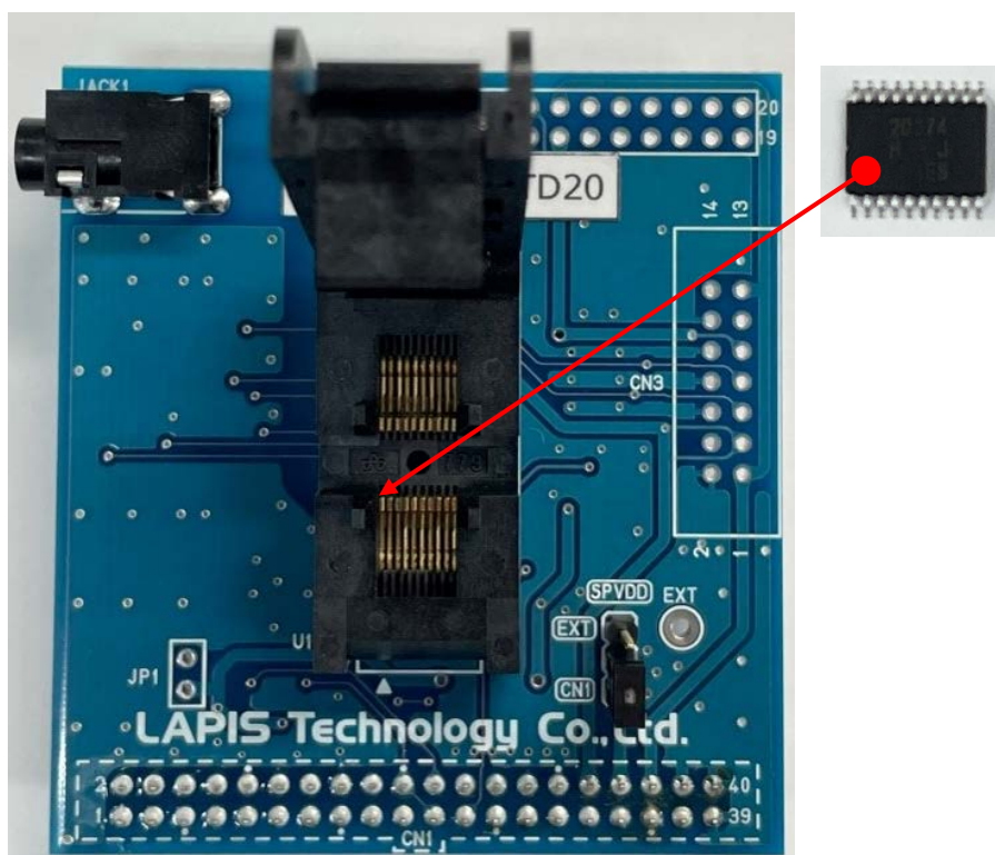
図 1 外観
