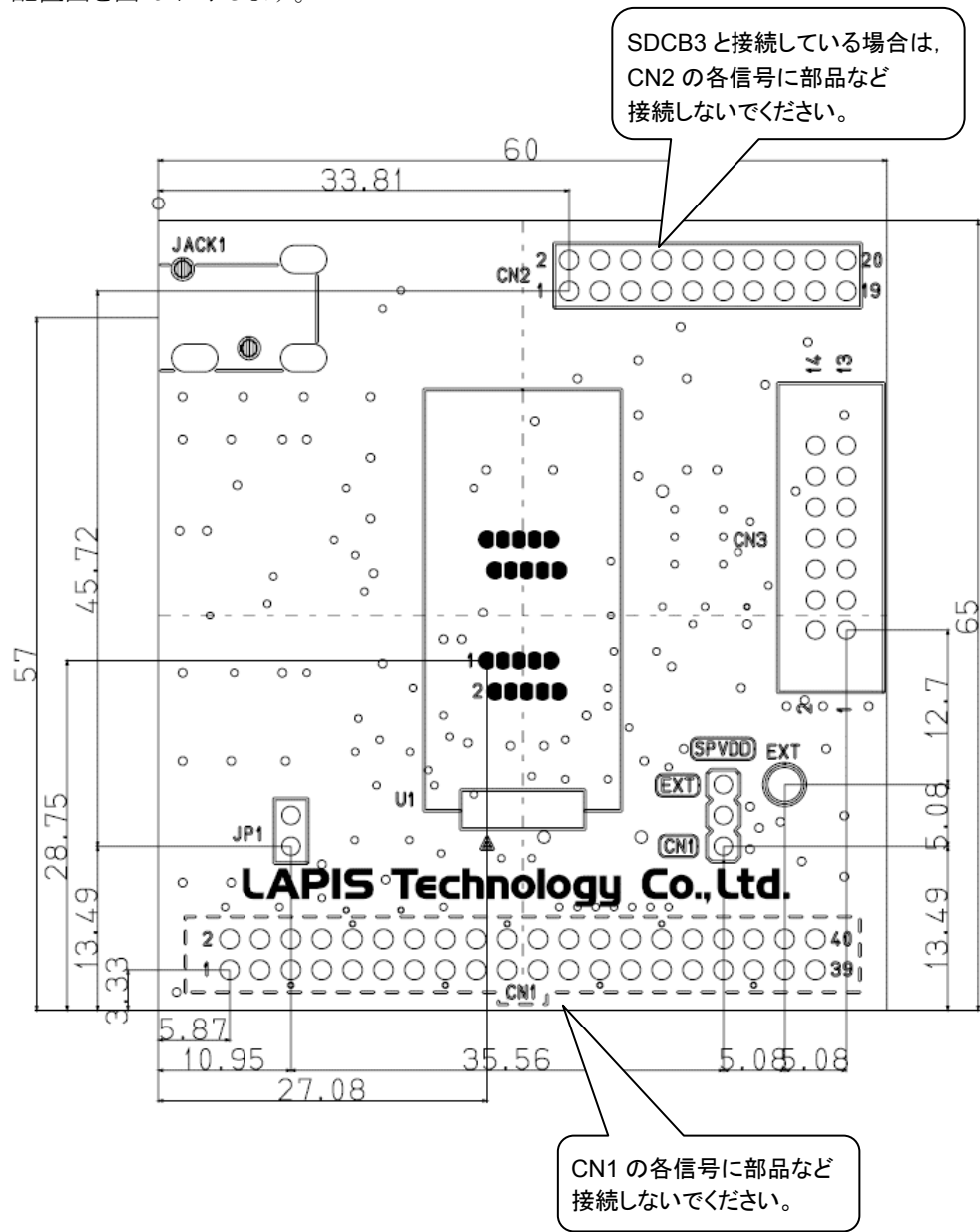
図 5 配置図
