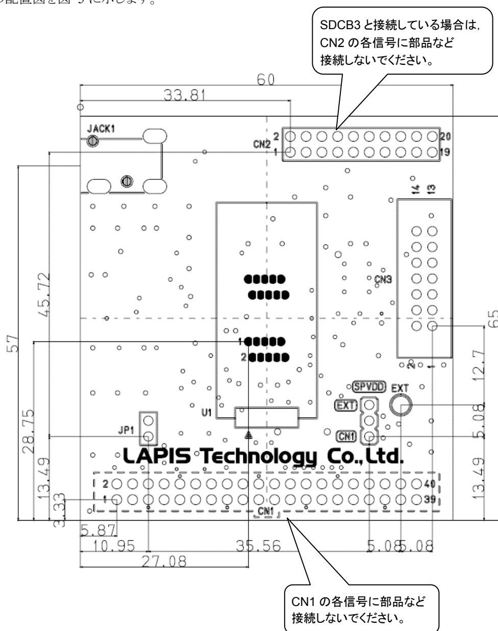
図 5 配置図
