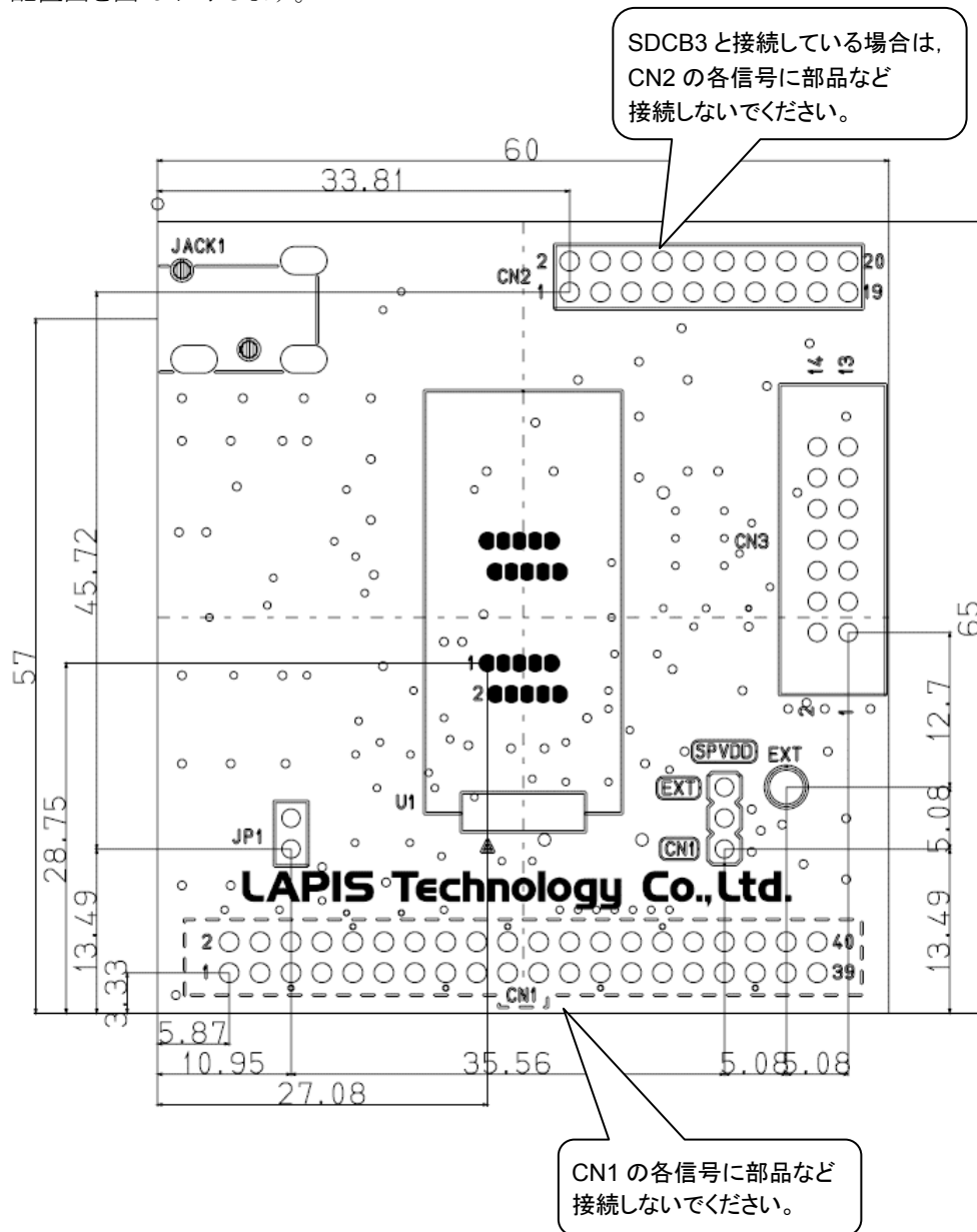
図 5 配置図
